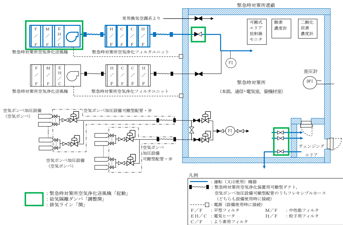
図 3-6 緊急時対策所換気空調系等の概要系統図（放射性雲通過前及び通過後）
