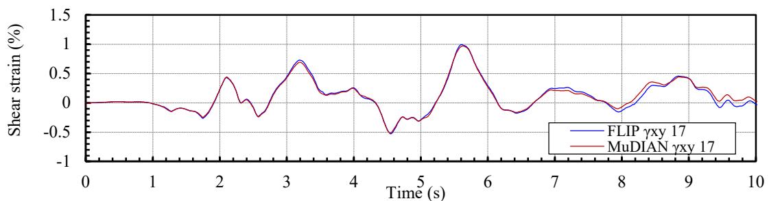
第 3.5.1-7 図 地盤のせん断ひずみ (時刻歴)
