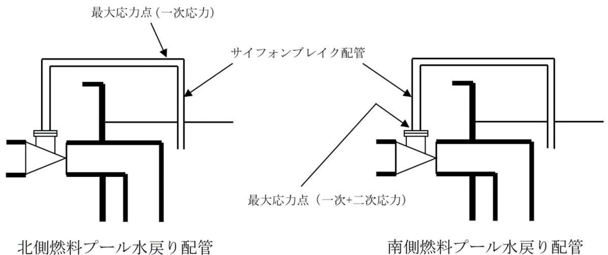
図6-1 最大応力点位置
