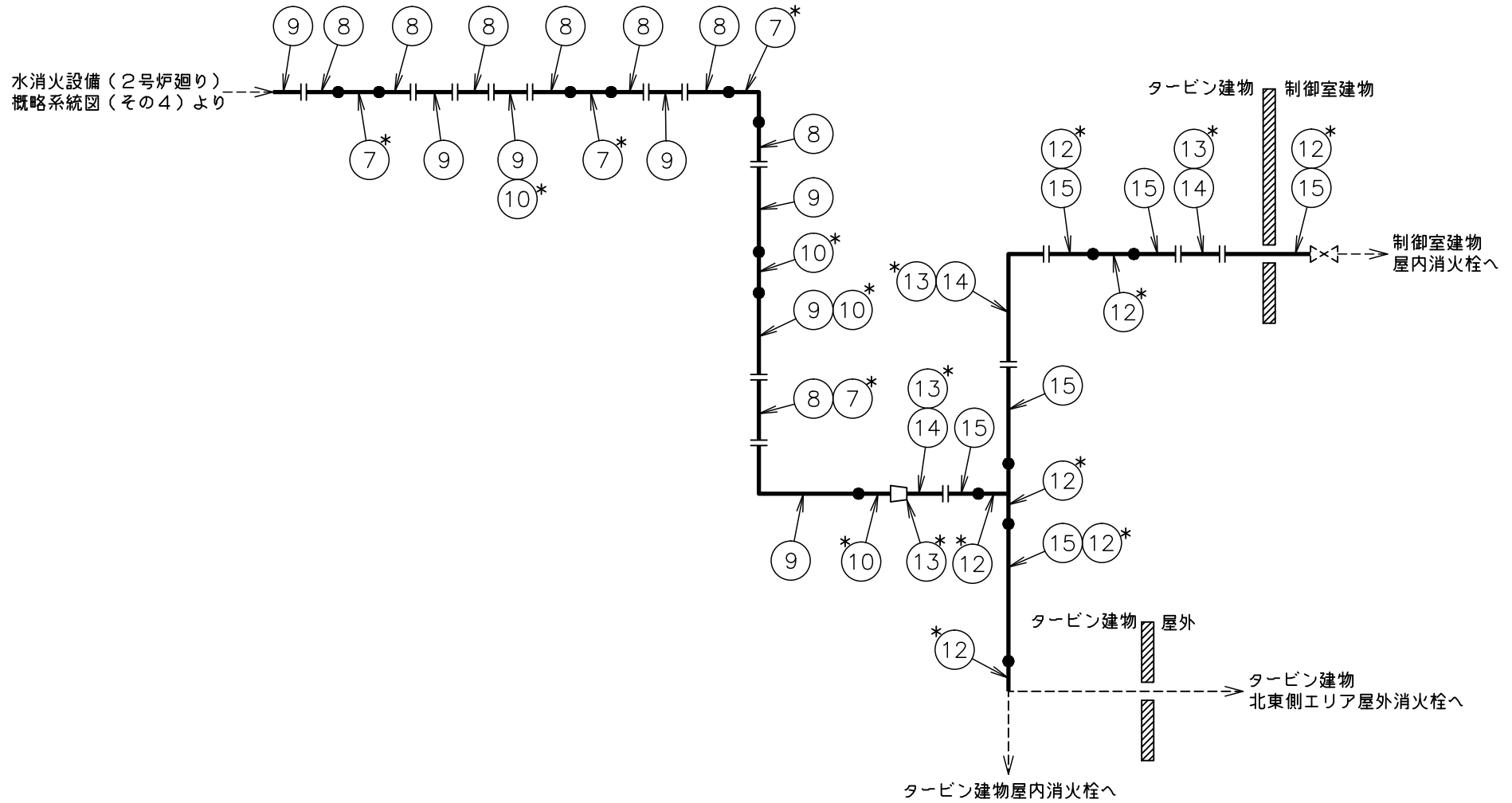
注記* : 管継手 水消火設備 (2号炉廻り) 概略系統図 (その5)
