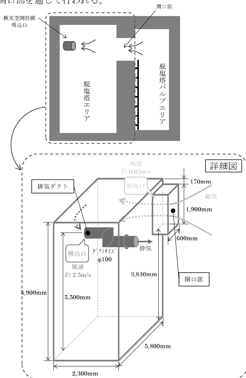
第 7-12 図 脱塩塔エリアの詳細図 (例：A,B 使用済燃料ピット脱塩塔エリア)
