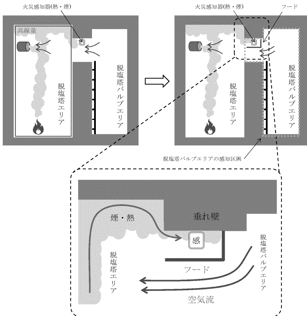
第 7-13 図 脱塩塔エリア開口部におけるフードを用いた火災感知器の設置概要
