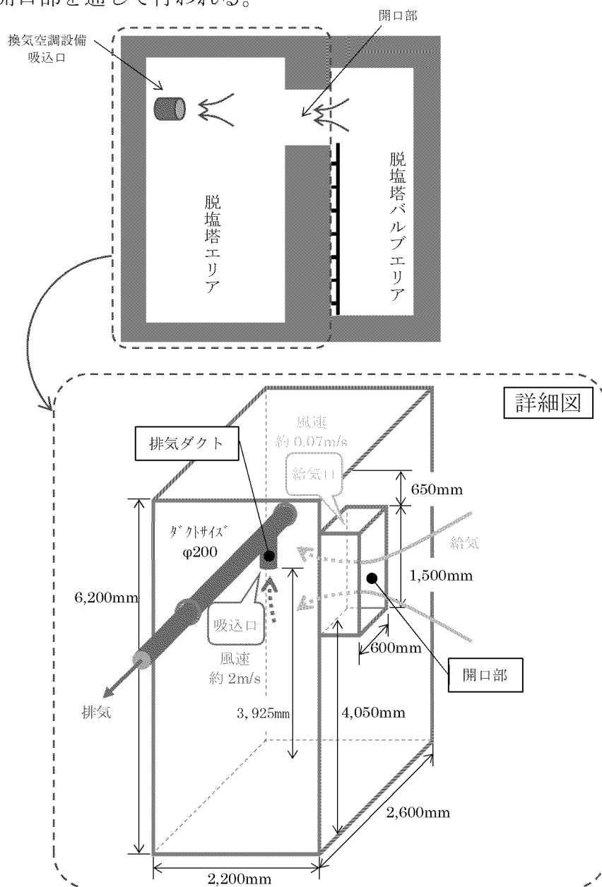
第 7-12 図 脱塩塔エリアの詳細図 (例：A 使用済燃料ピット脱塩塔エリア)
