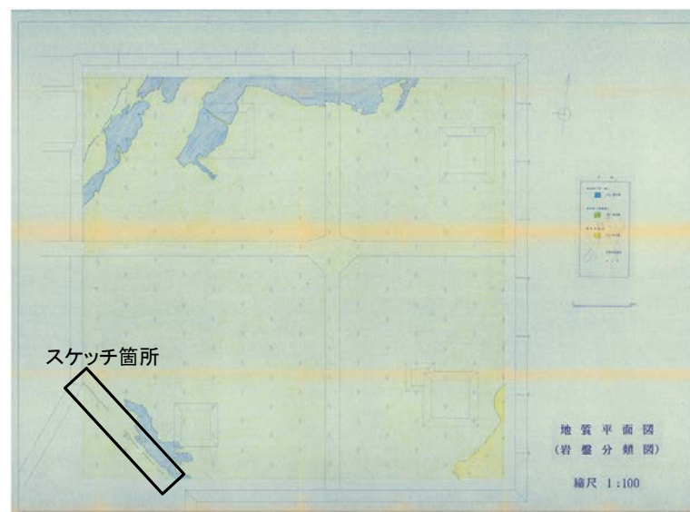
1号機基礎掘削面(EL-7.1m) 地質平面図
