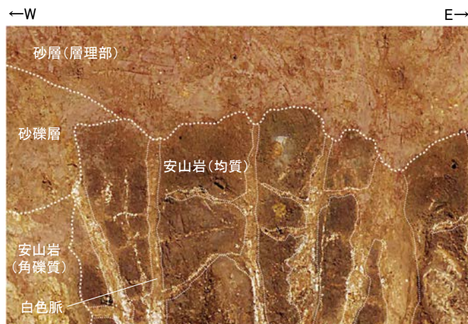
白色脈と第四系との関係 拡大写真(大坪川ダム右岸トレンチ)
