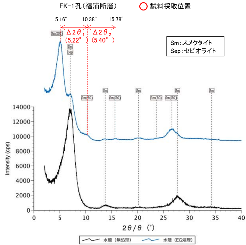
X線回折チャート(定方位)
