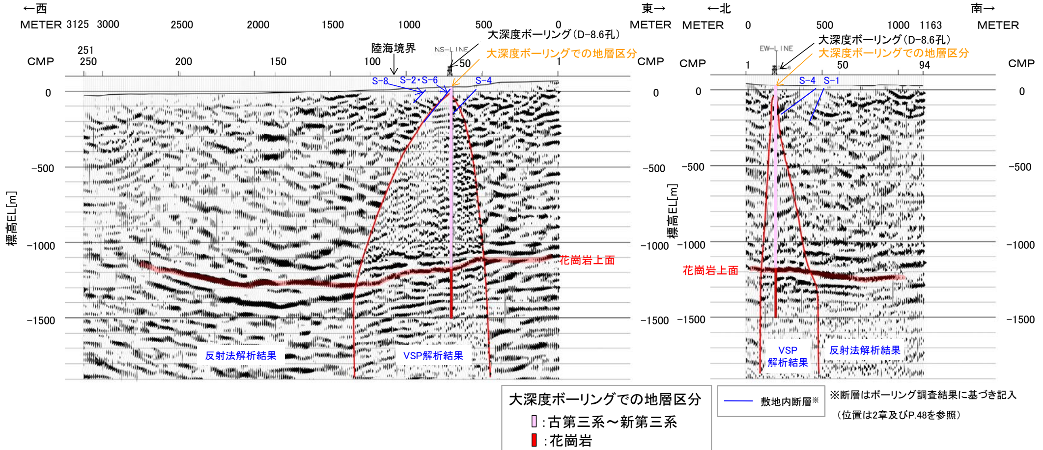
反射法・VSP探査結果(南北測線:深度断面)
