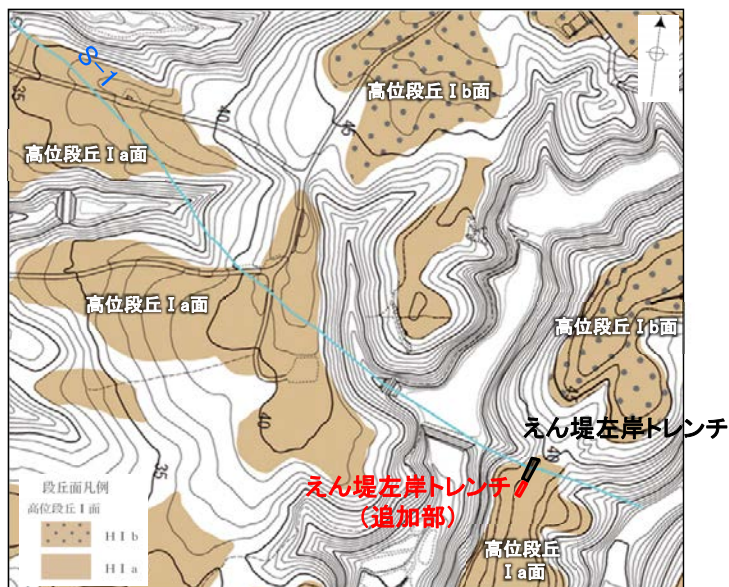
断層(地表に投影) トレンチ 0 200m
