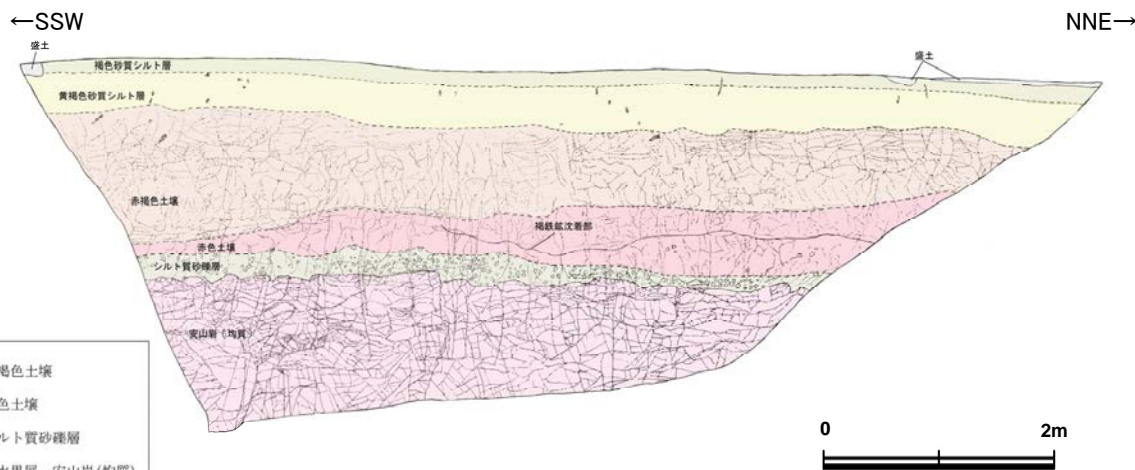
スケッチ(西壁面)
