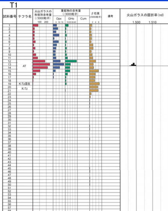
試料は5cm間隔 ■パフルウォール混タイプ Opqx:斜方輝石 GHo:緑色普通角閃石 Cum:カランタン閃石
