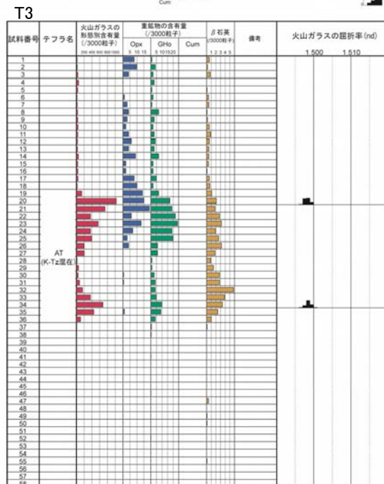
試料は5cm間隔 ■パフルウォール混タイプ Opqx:斜方輝石 GHo:緑色普通角閃石 Cum:カランタン閃石
