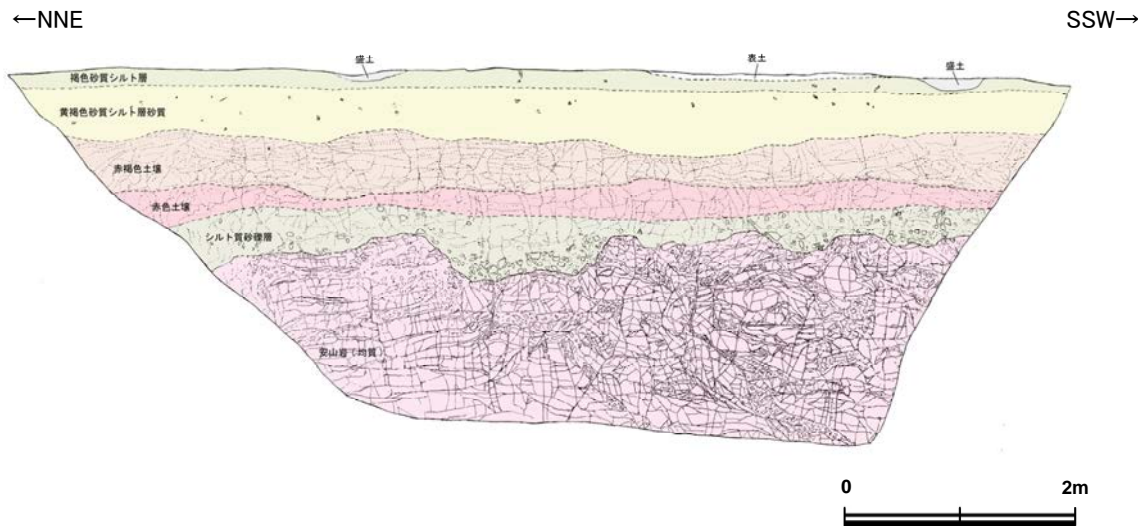
スケッチ(東壁面)
