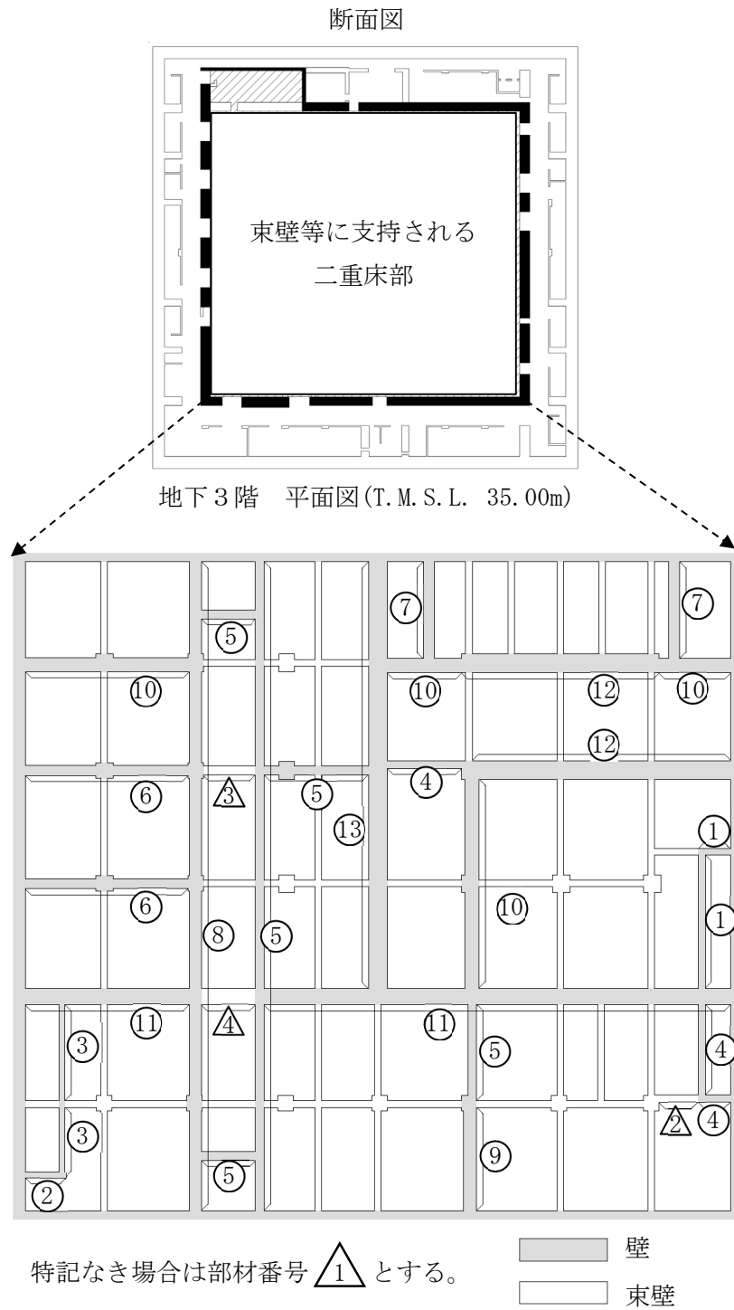
第 3.2-2 図 東壁部及び壁の部材リスト (T.M.S.L. 34.23m~34.40m)
