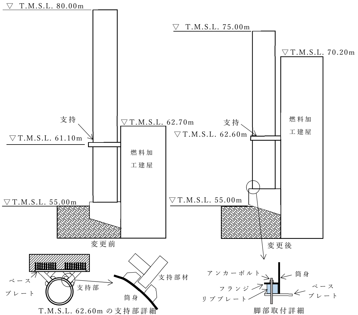
第 2.2.1-2 図 設計変更前後の排気筒と燃料加工建屋との取り合い
