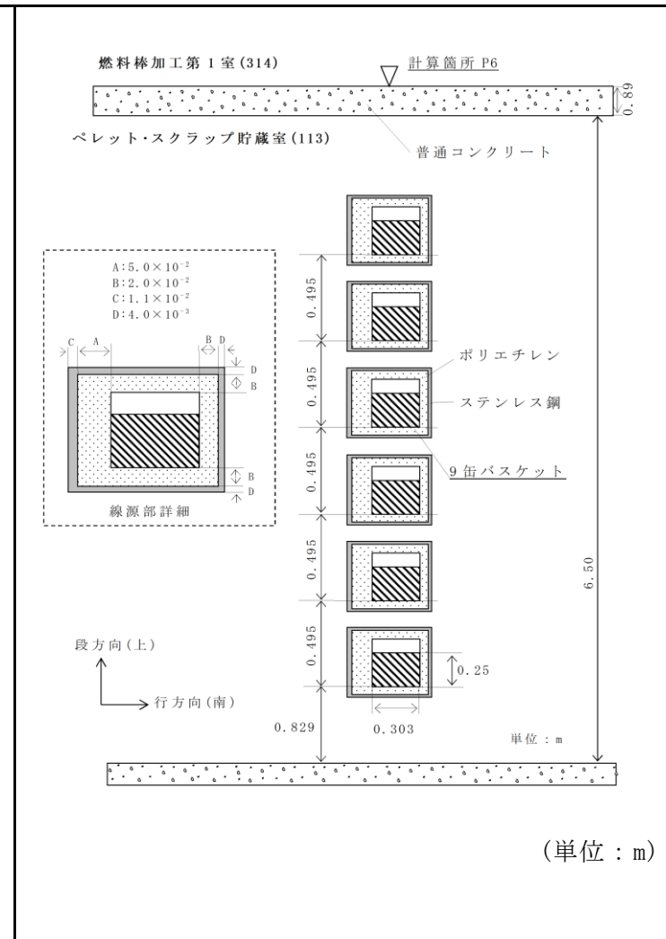
計算モデル(2次元無限角柱モデル)
