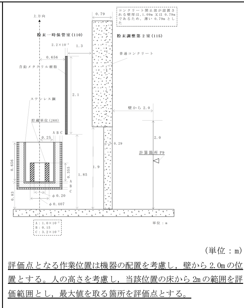
計算モデル(2次元円筒モデル)
