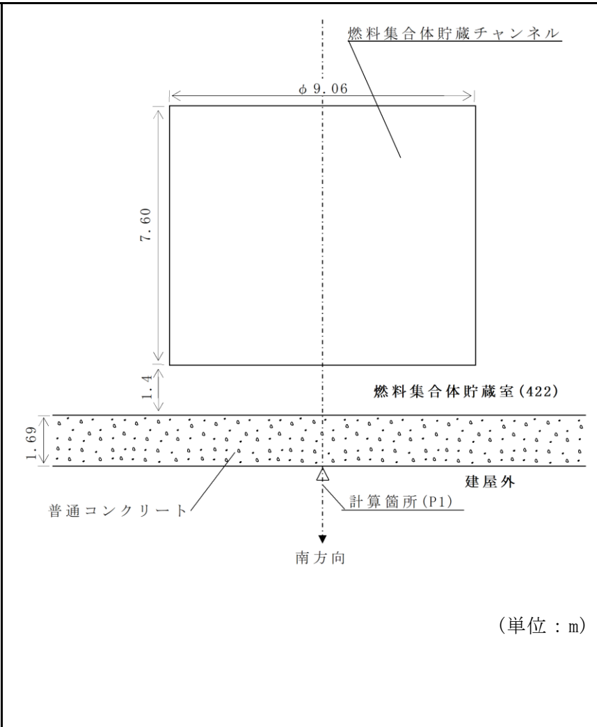
計算モデル(2次元円筒モデル)
