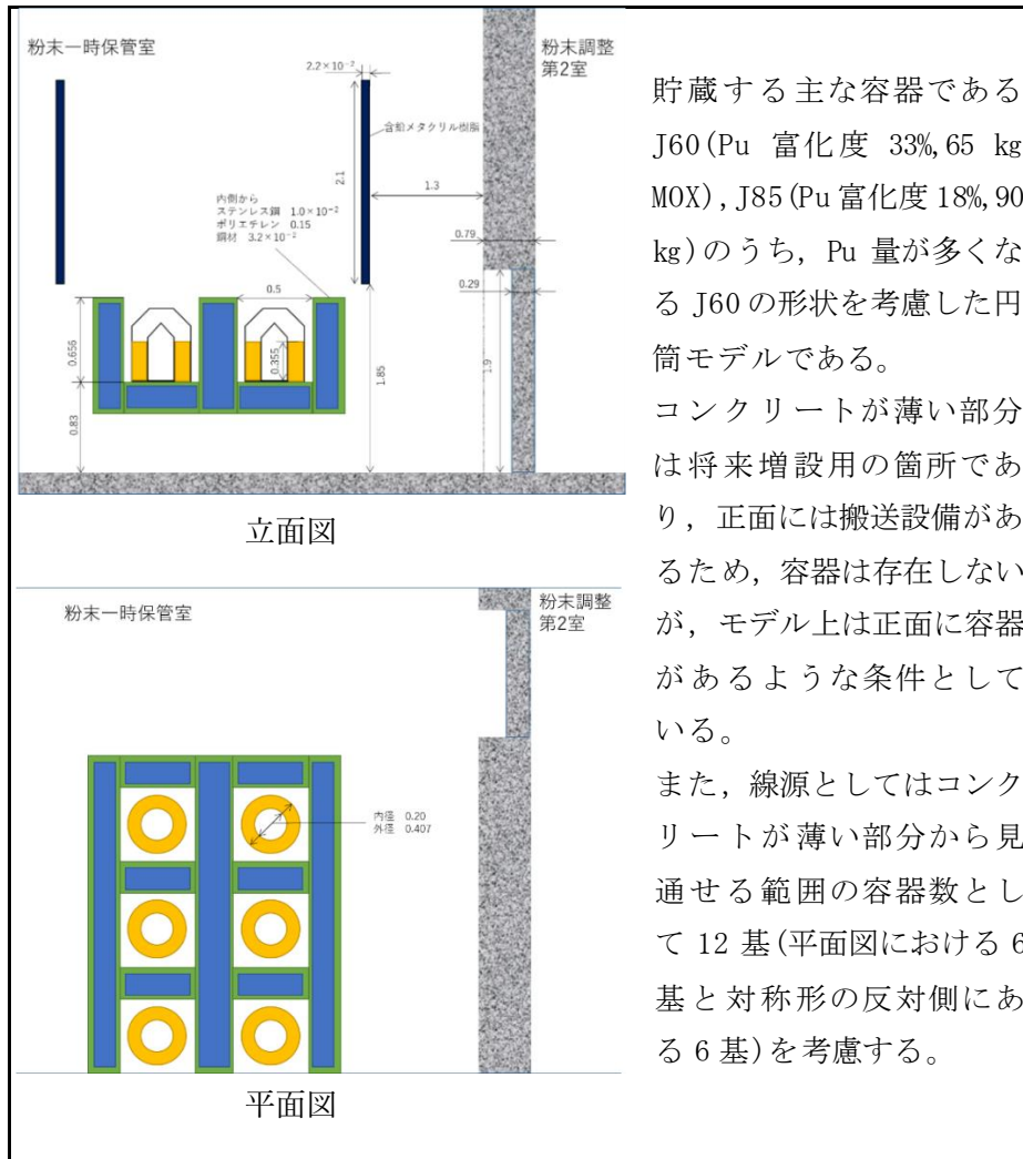
概要図
