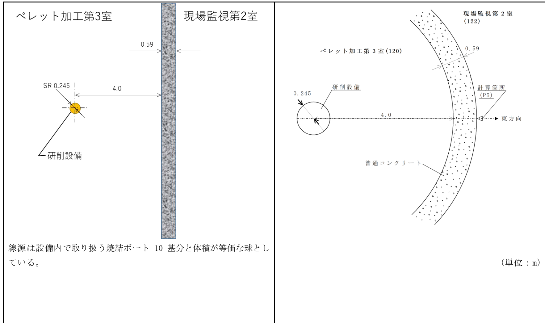
概要図
