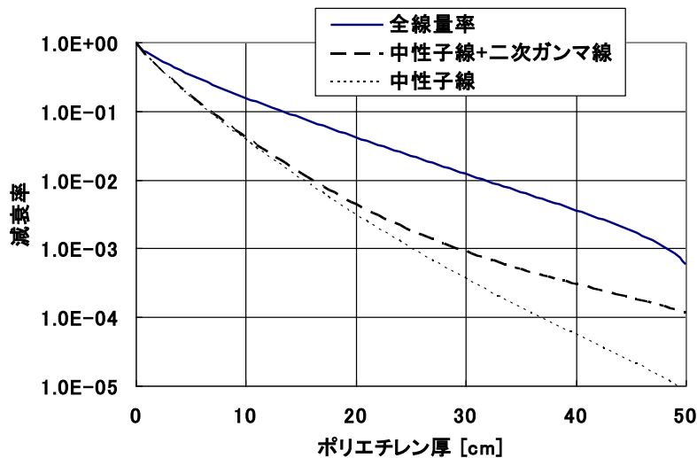
第 3.3-1 図 ポリエチレン厚さと減衰率
