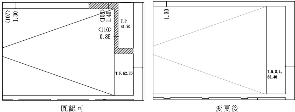
第 3.2.3-1 図 建屋遮蔽の変更(地上 2 階 輸送容器保管室北東部抜粋)
