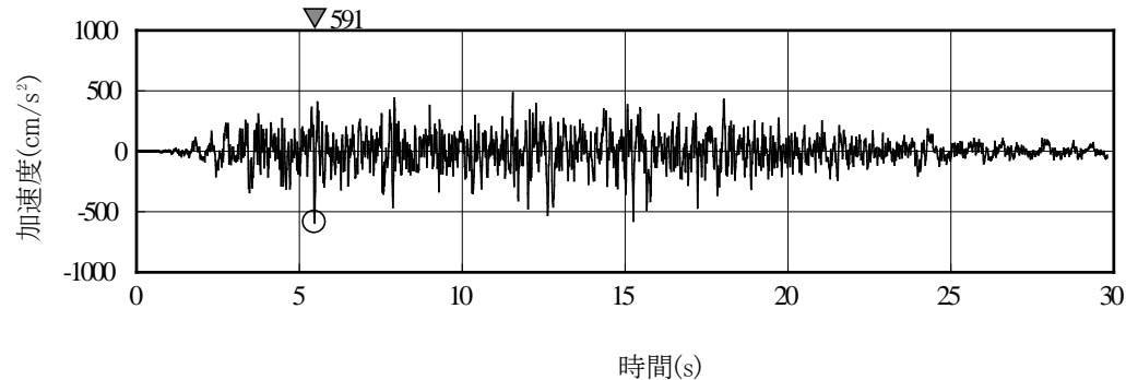
鉛直成分
