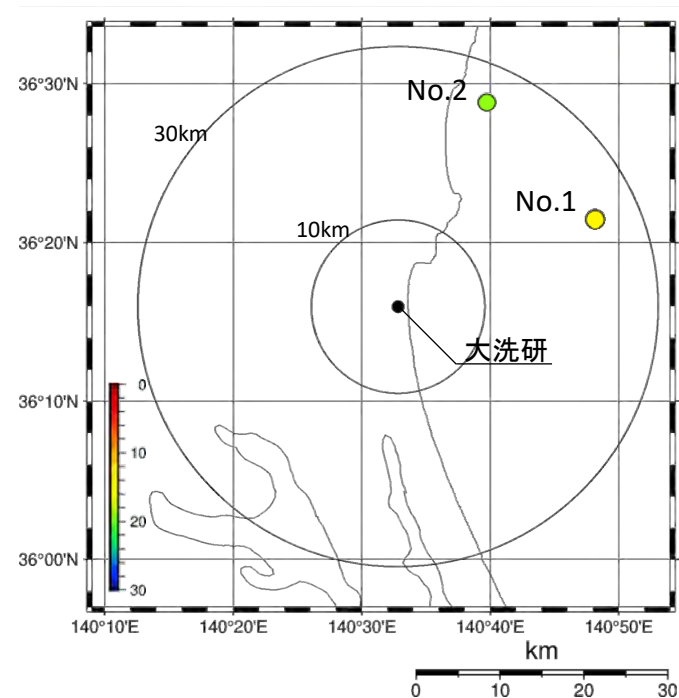
震央分布図
