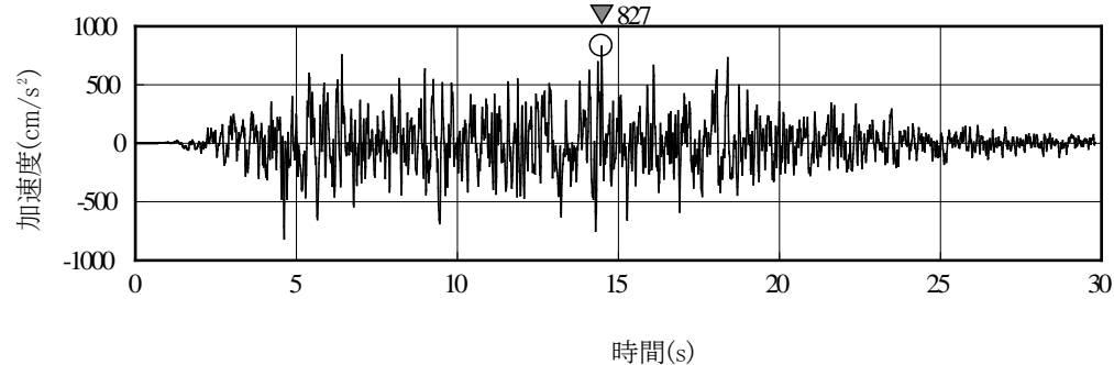
水平成分
