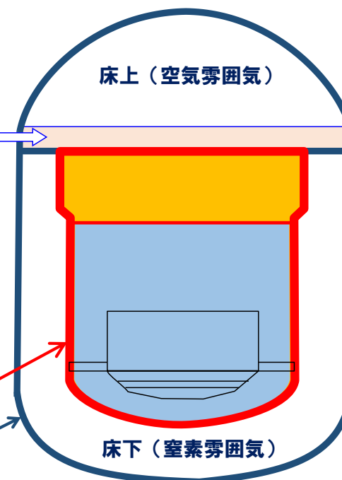
【概略系統図】
