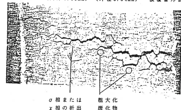
フィッシャー型破損の例 (EBR-II) *
