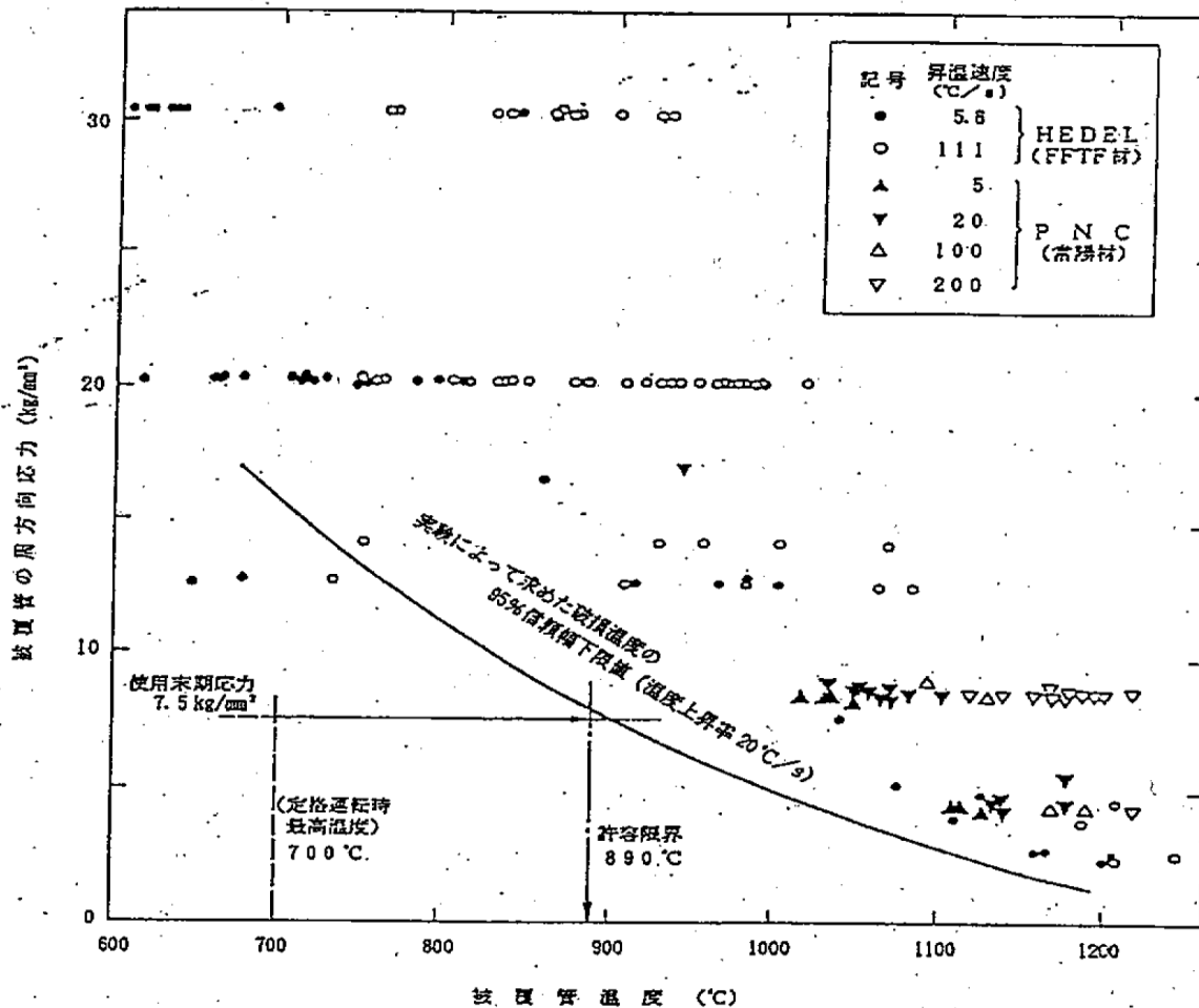
オーステナイト系ステンレス鋼の破損温度
