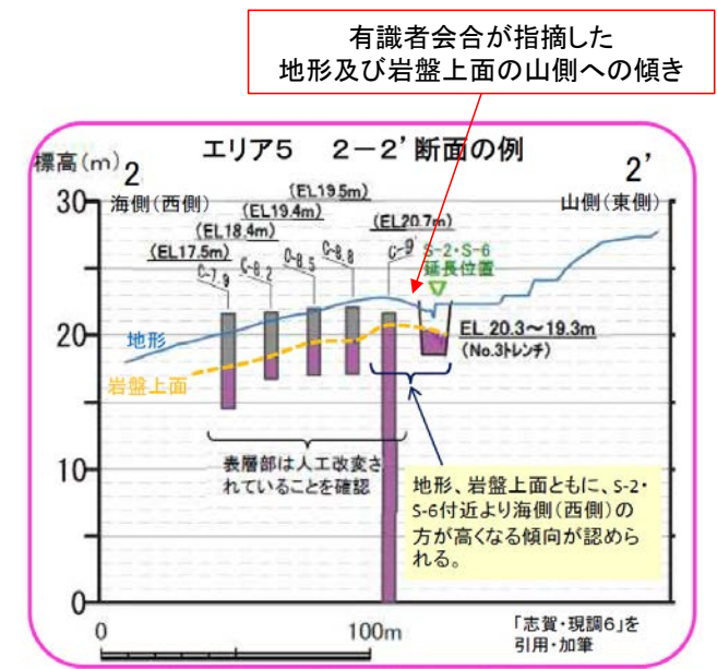
断面図
