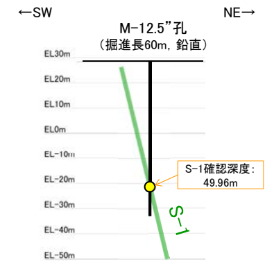
M-12.5"孔断面図 (断層直角方向, H:V=1:1)
