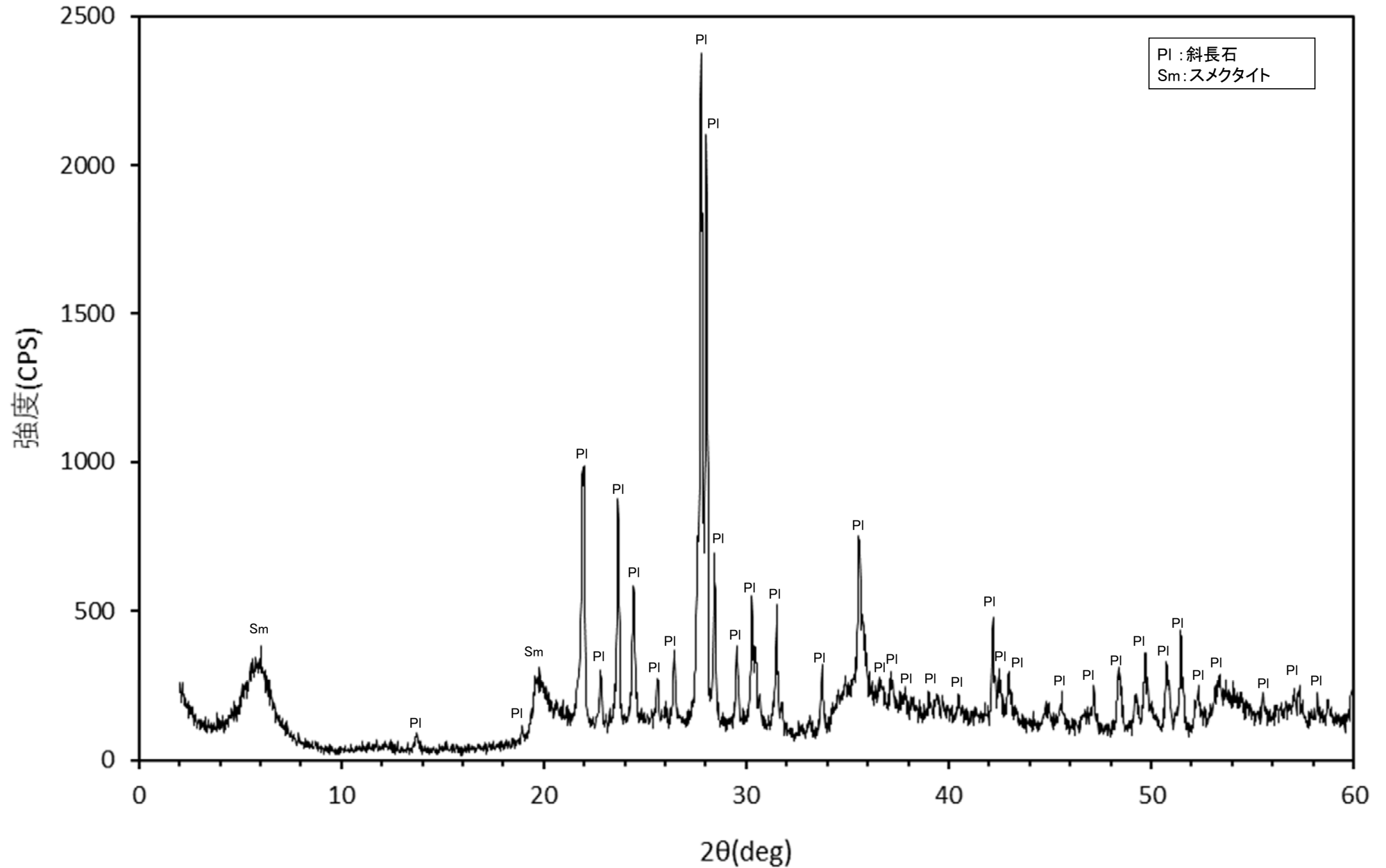
回折チャート
