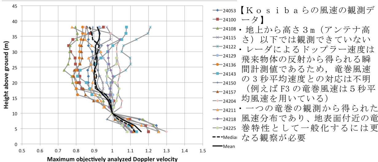
図 25 地上からの高さと同風速 (ドップラー速度) 分布 (6)
