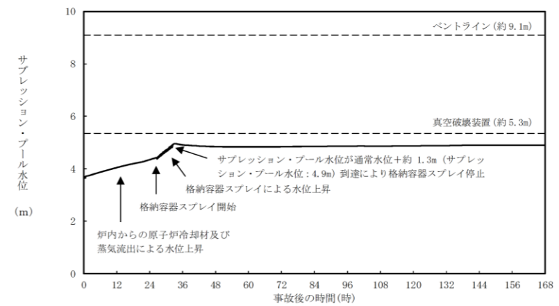
図 4-12 重大事故等時のサブプレッションプールの水位の変化*
