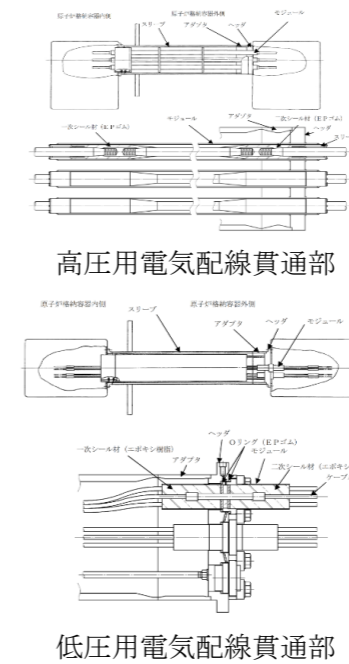
図 6-3 原子炉格納容器バウンダリ構造部概要図(5/6)
