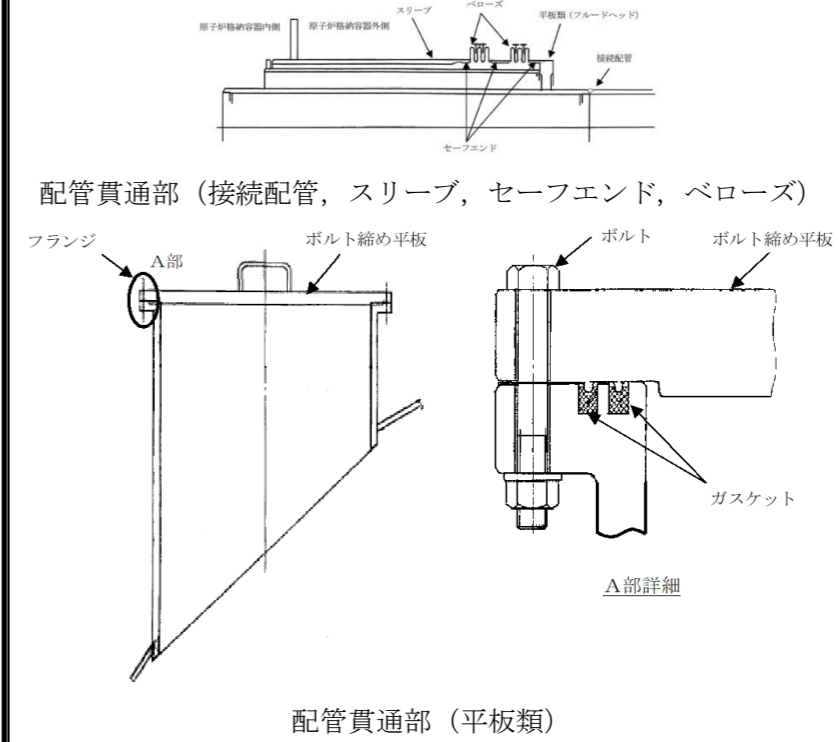
図 6-3 原子炉格納容器バウンダリ構造部概要図(4/6)
