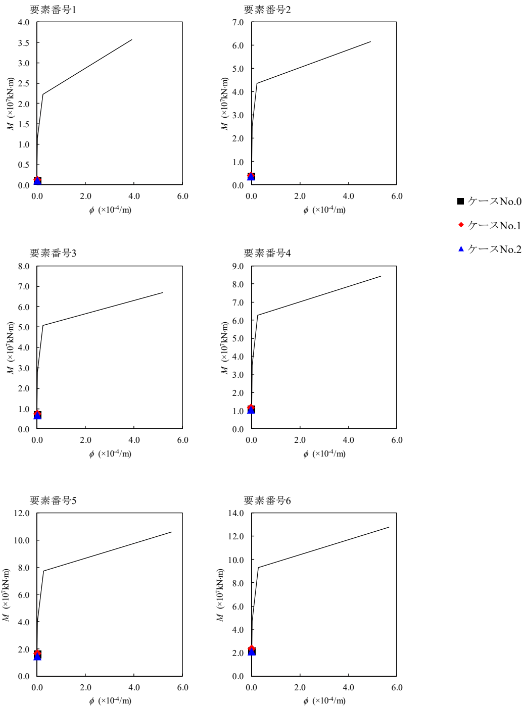
第 4.1.3-52 図 M-phi 関係と最大応答値 (S d - B 3, EW 方向)
