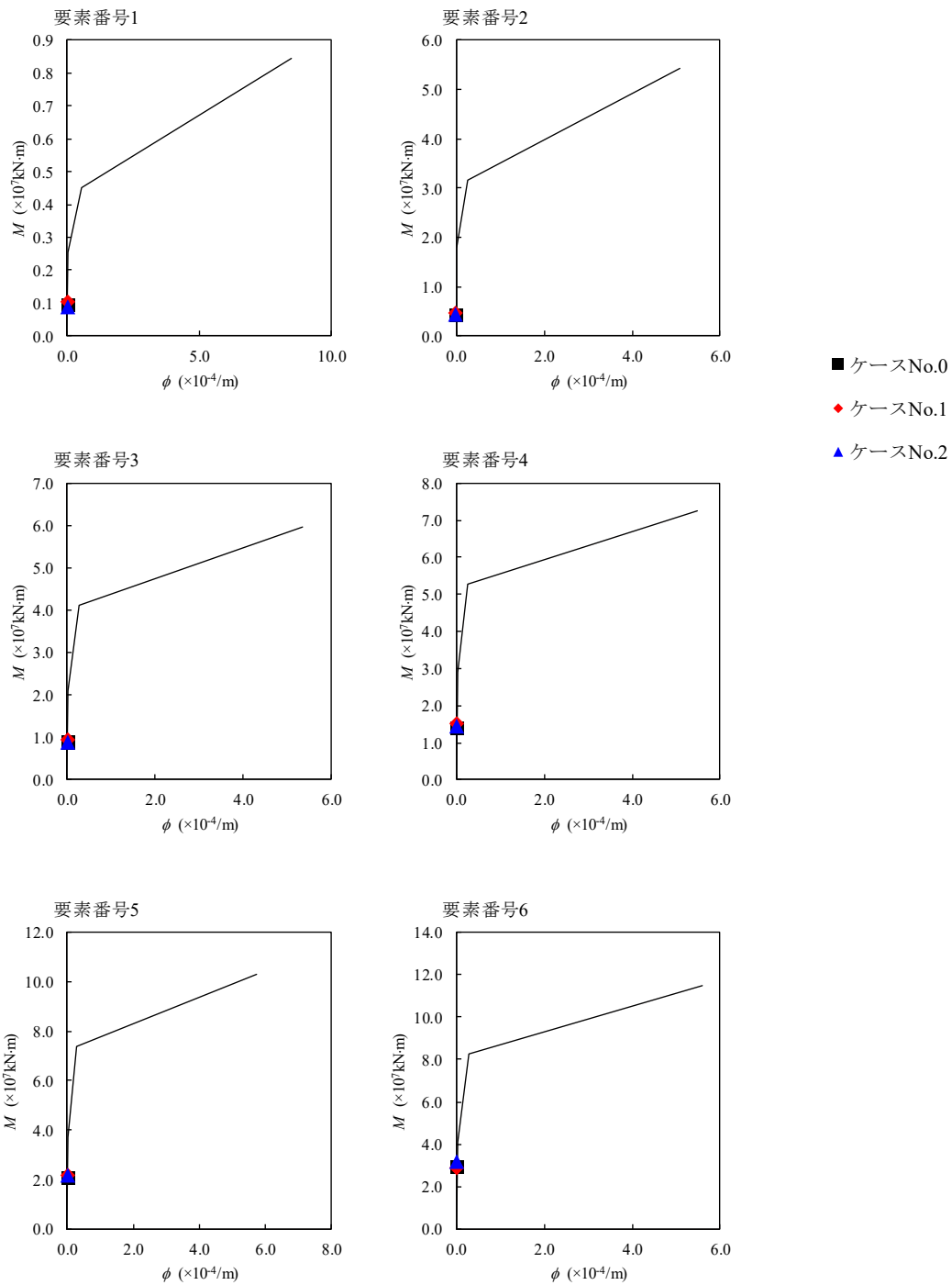
第 4.1.3-40 図 M-φ 関係と最大応答値 (S d - A, NS 方向)
