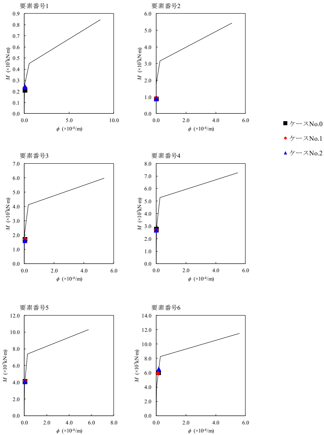
第 4.1.3-19 図 M- \phi 関係と最大応答値 (S s -C1, NS 方向)
