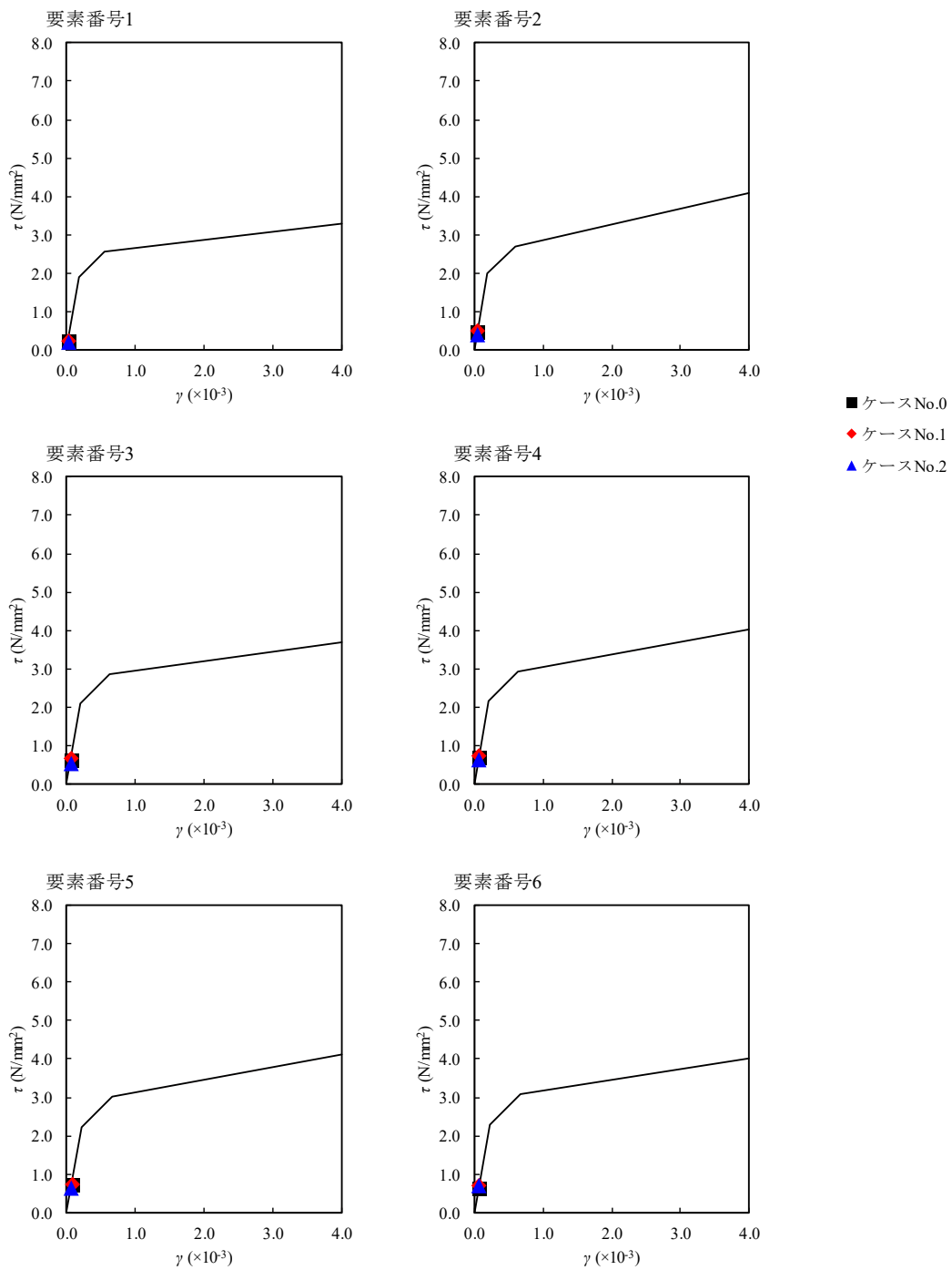
第 4.1.3-51 図 \tau - \gamma 関係と最大応答値 (S d - B 3, EW 方向)
