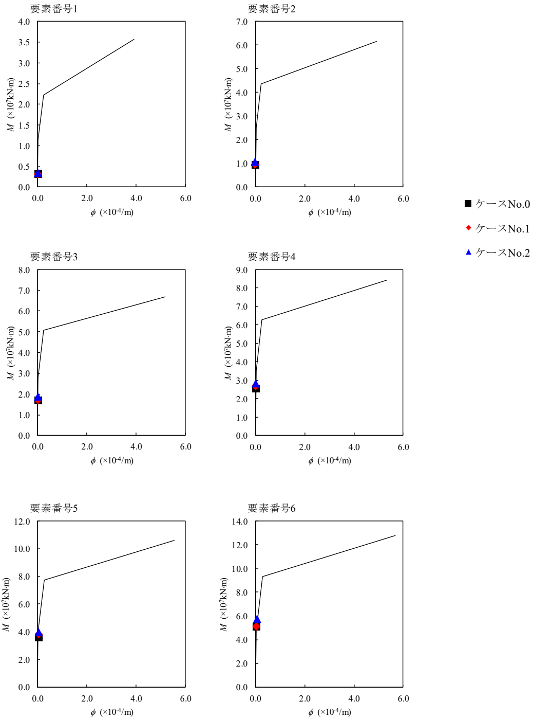
第 4.1.3-21 図 M-φ 関係と最大応答値 (S s -A, EW 方向)
