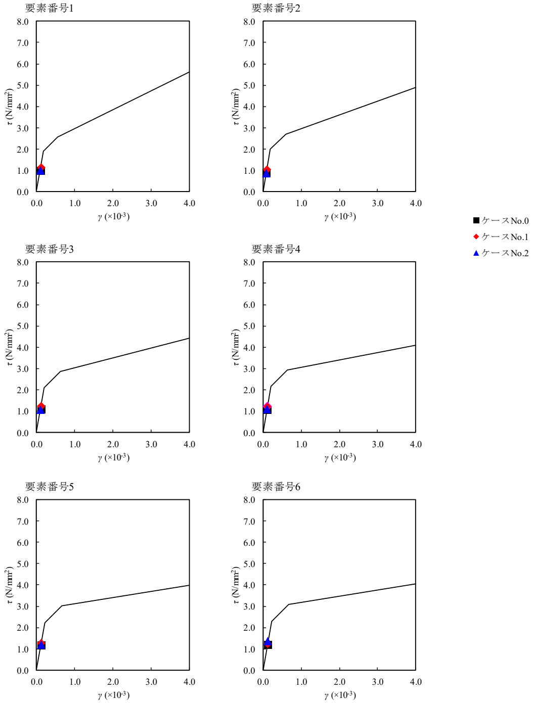
第 4.1.3-14 図 \tau - \gamma 関係と最大応答値 (S s -B1, NS 方向)
