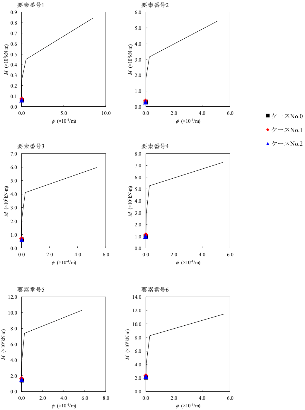
第 4.1.3-44 図 M-φ 関係と最大応答値 (S d - B 3, NS 方向)
