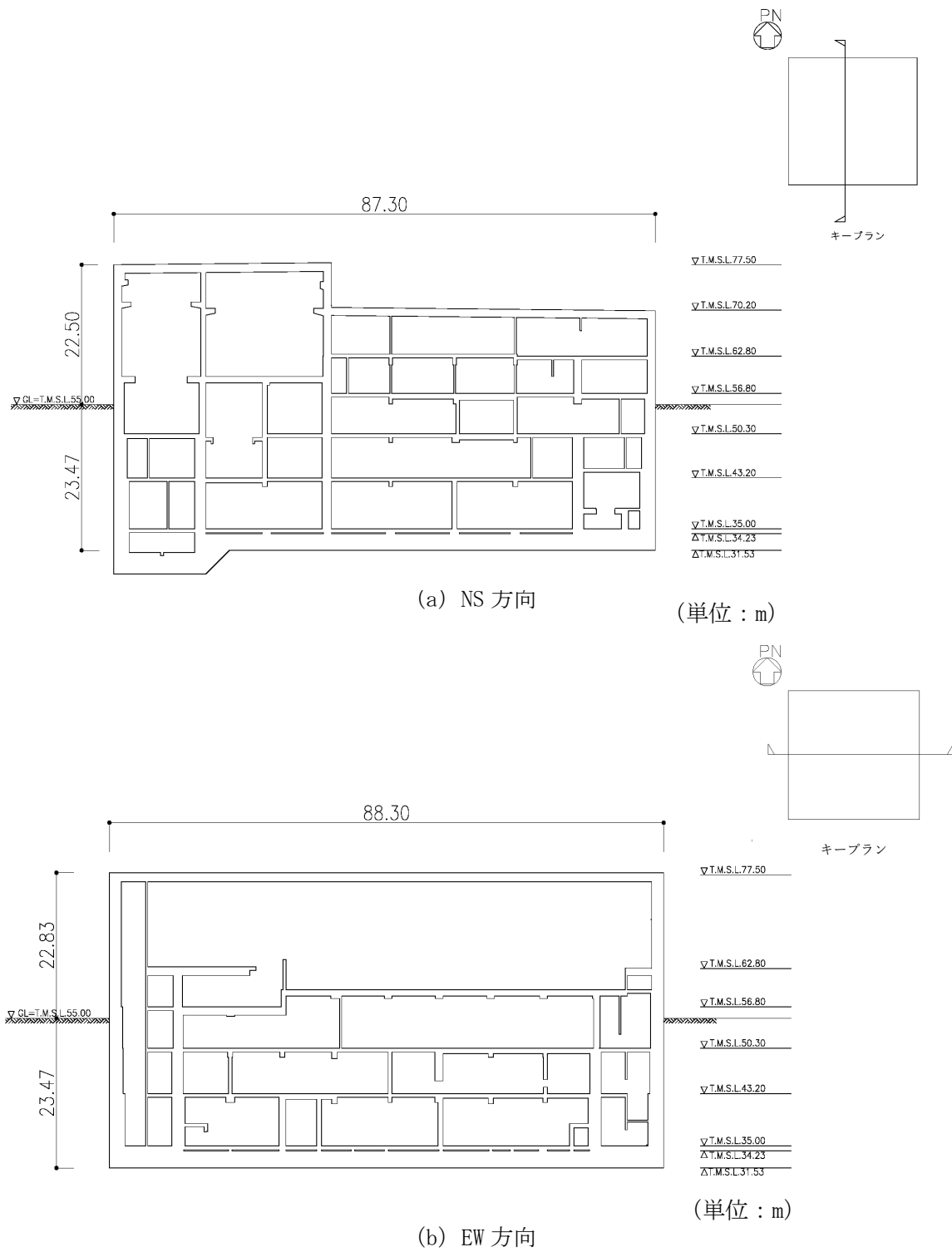
第 2.2-2 図 概略断面図
