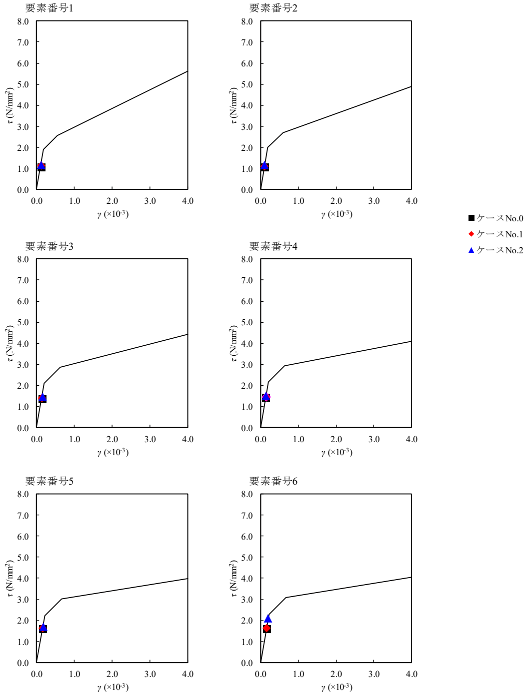
第 4.1.3-16 図 \tau - \gamma 関係と最大応答値 (S s - B 3, NS 方向)
