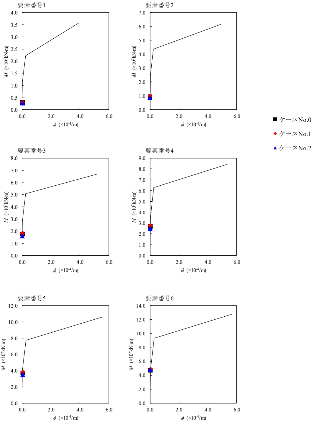
第 4.1.3-23 図 M-φ 関係と最大応答値 (S s -B1, EW 方向)
