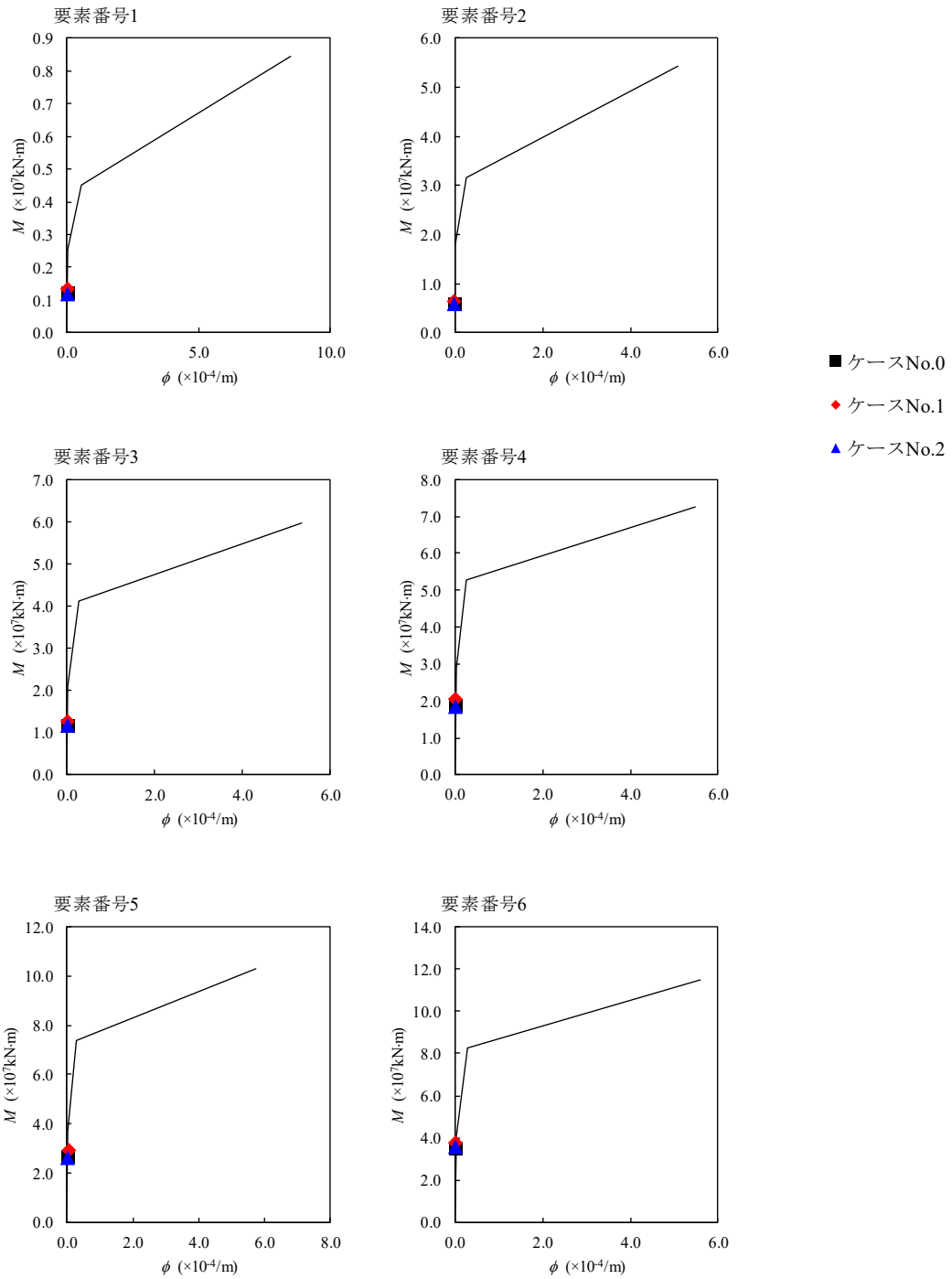
第 4.1.3-15 図 M- \phi 関係と最大応答値 (S s -B1, NS 方向)
