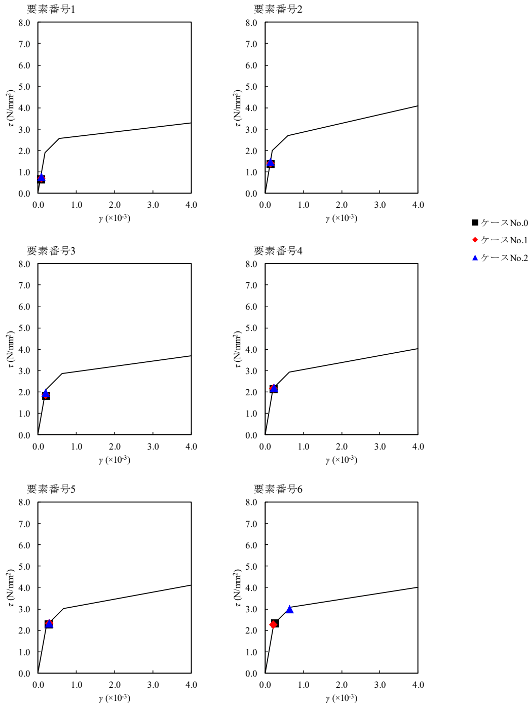
第 4.1.3-26 図 \tau - \gamma 関係と最大応答値 (S s - C 1, EW 方向)
