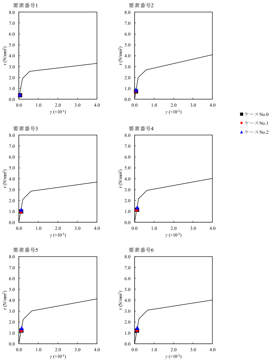
第 4.1.3-53 図 \tau - \gamma 関係と最大応答値 (S d - C 1, EW 方向)
