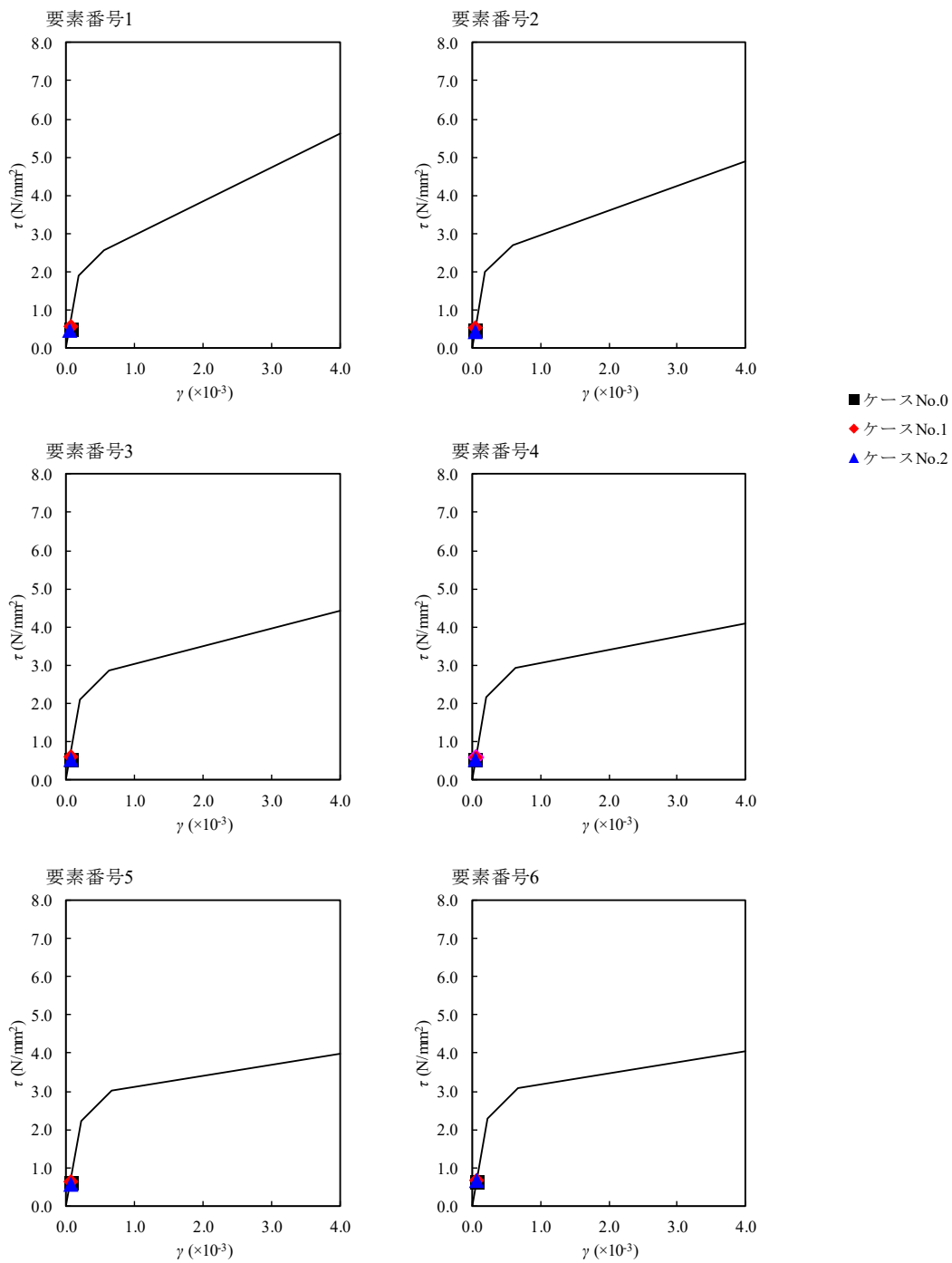
第 4.1.3-43 図 \tau - \gamma 関係と最大応答値 (S d - B 3, NS 方向)
