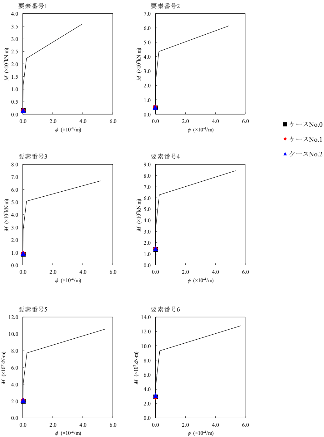
第 4.1.3-48 図 M-phi 関係と最大応答値 (S d - A, EW 方向)
