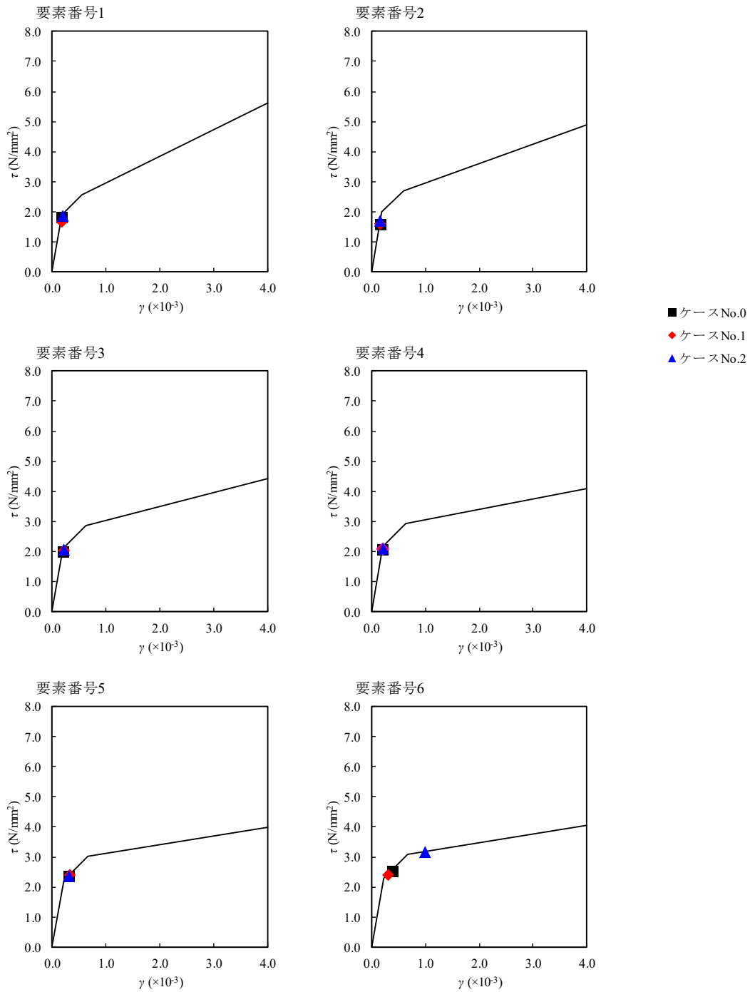
第 4.1.3-18 図 \tau - \gamma 関係と最大応答値 (S s -C1, NS 方向)
