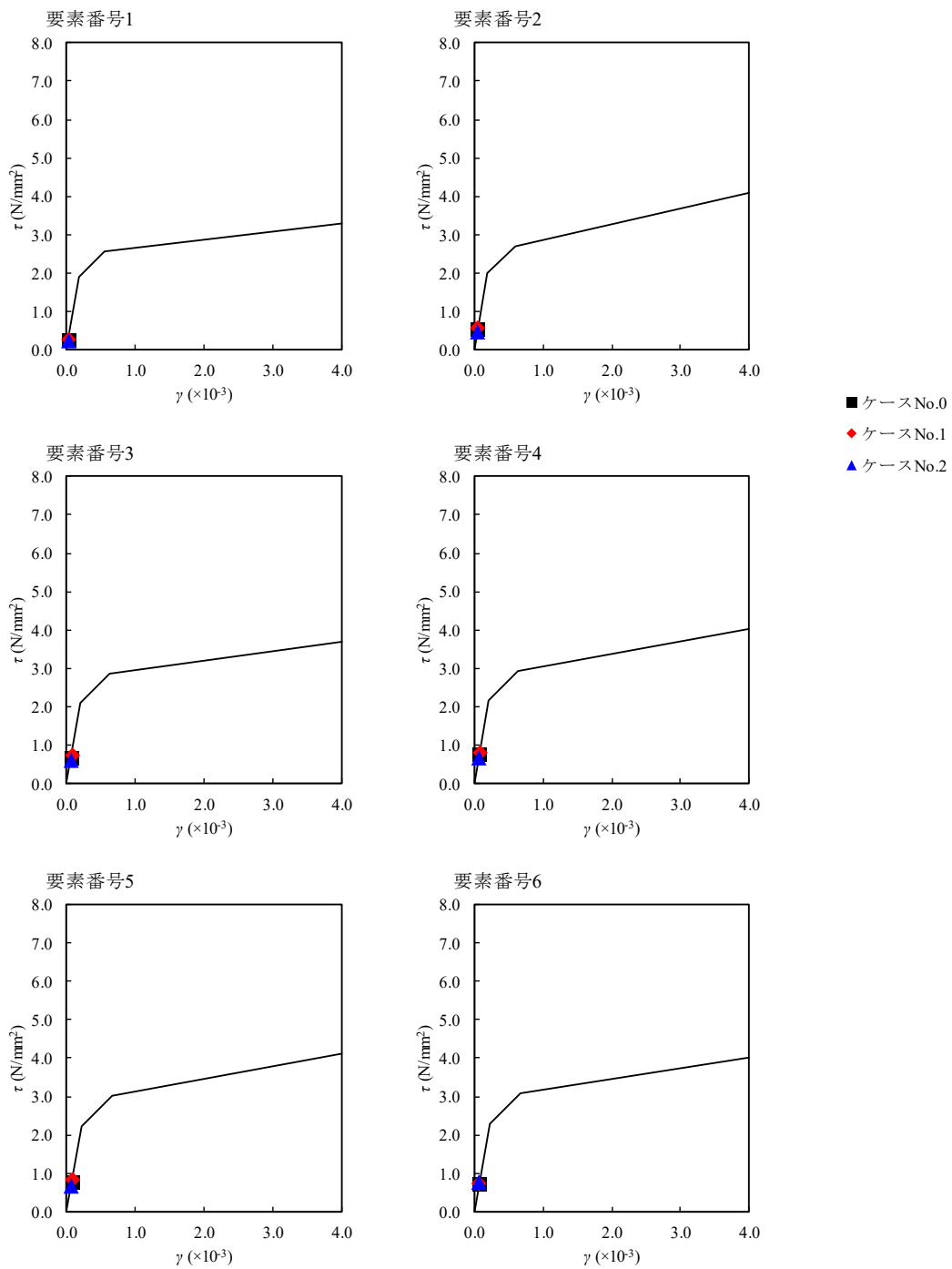
第 4.1.3-49 図 \tau - \gamma 関係と最大応答値 (S d - B 1, EW 方向)
