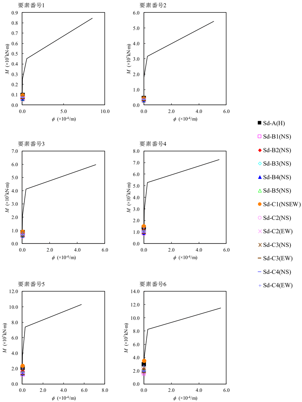
第4.1.2-28 図 M-φ関係と最大応答値 (弾性設計用地震動S d , ケースNo.0, NS方向)
