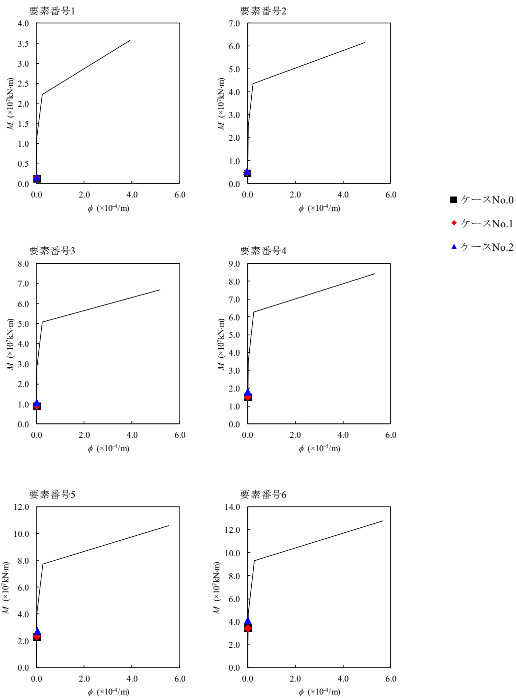
第 4.1.3-54 図 M-φ 関係と最大応答値 (S d - C 1, EW 方向)
