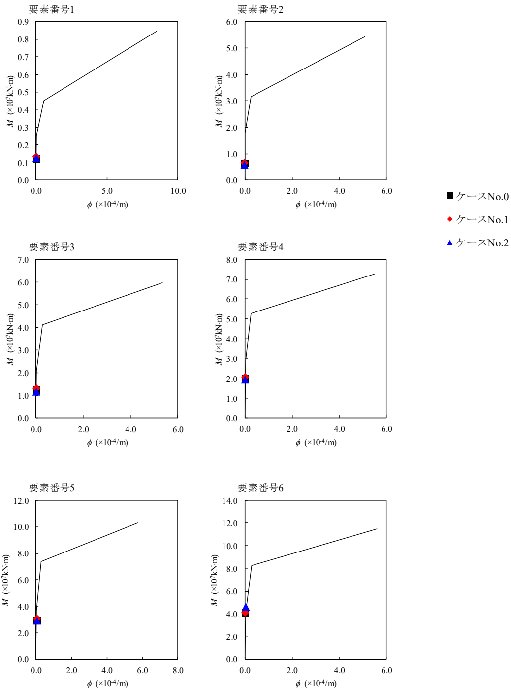
第 4.1.3-17 図 M-φ 関係と最大応答値 (S s - B 3, NS 方向)
