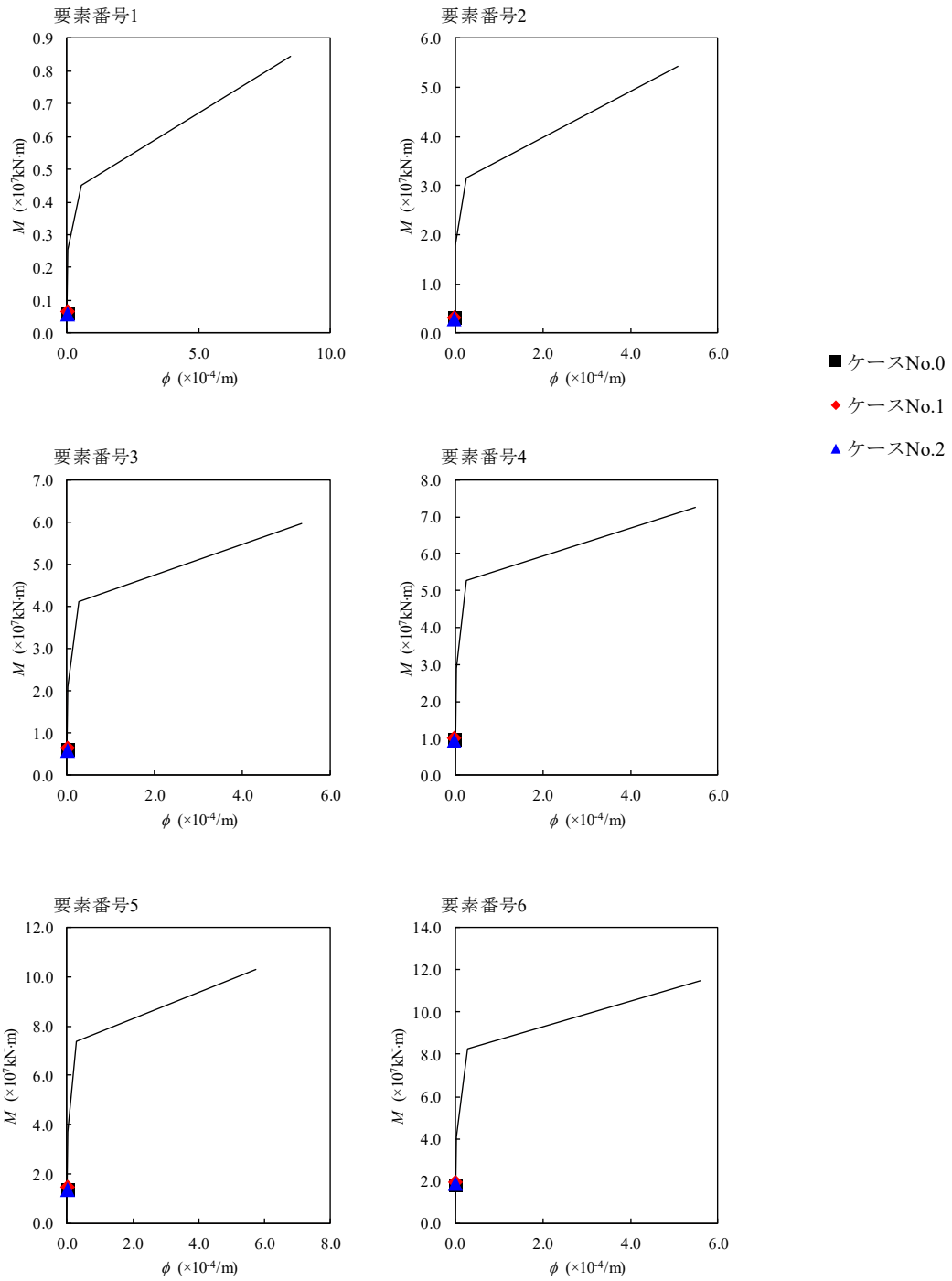
第 4.1.3-42 図 M-φ 関係と最大応答値 (S d - B 1, NS 方向)
