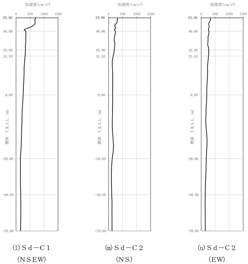
第 3. 3. 1-7 図 最大加速度分布 (4/5) (S d)
