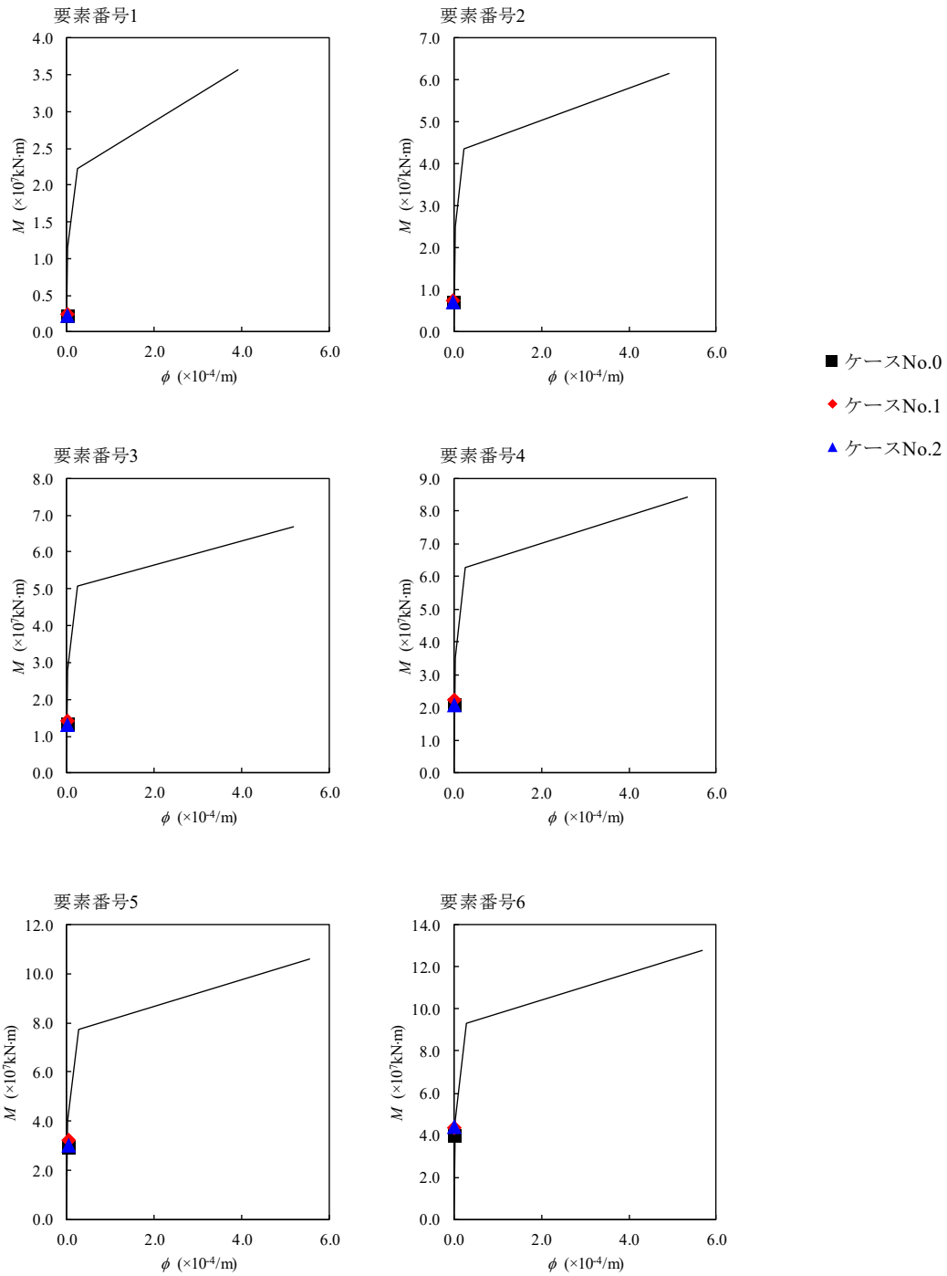
第 4.1.3-25 図 M-φ 関係と最大応答値 (S s -B3, EW 方向)
