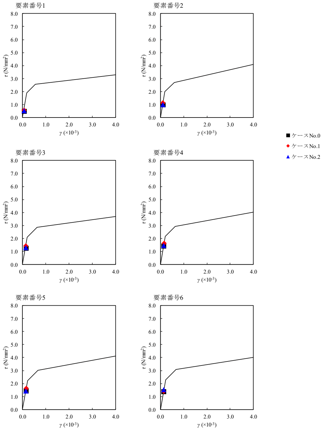
第 4.1.3-22 図 \tau - \gamma 関係と最大応答値 (S s -B1, EW 方向)
