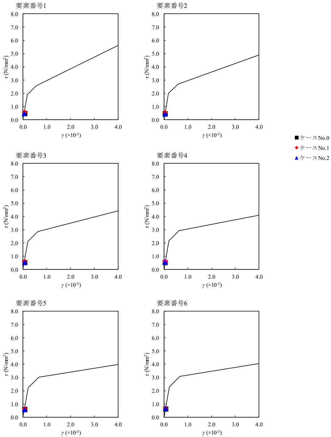
第 4.1.3-41 図 \tau - \gamma 関係と最大応答値 (S d - B 1, NS 方向)
