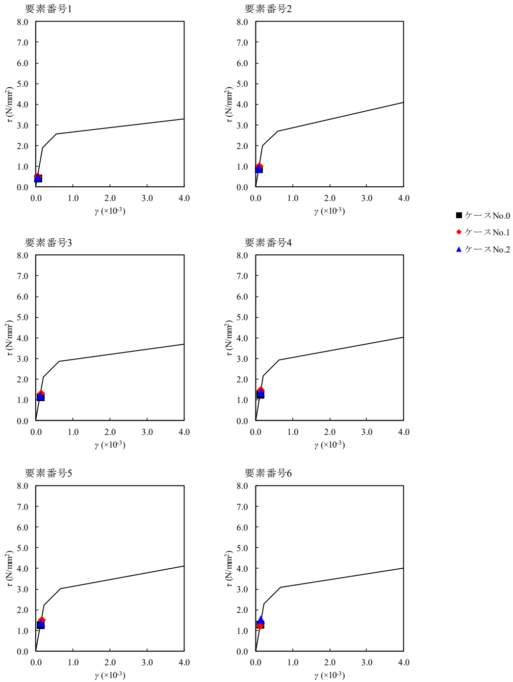
第 4.1.3-24 図 \tau - \gamma 関係と最大応答値 (S s - B 3, EW 方向)
