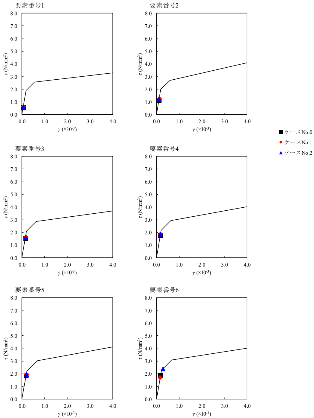
第 4.1.3-20 図 \tau - \gamma 関係と最大応答値 (S s - A, EW 方向)
