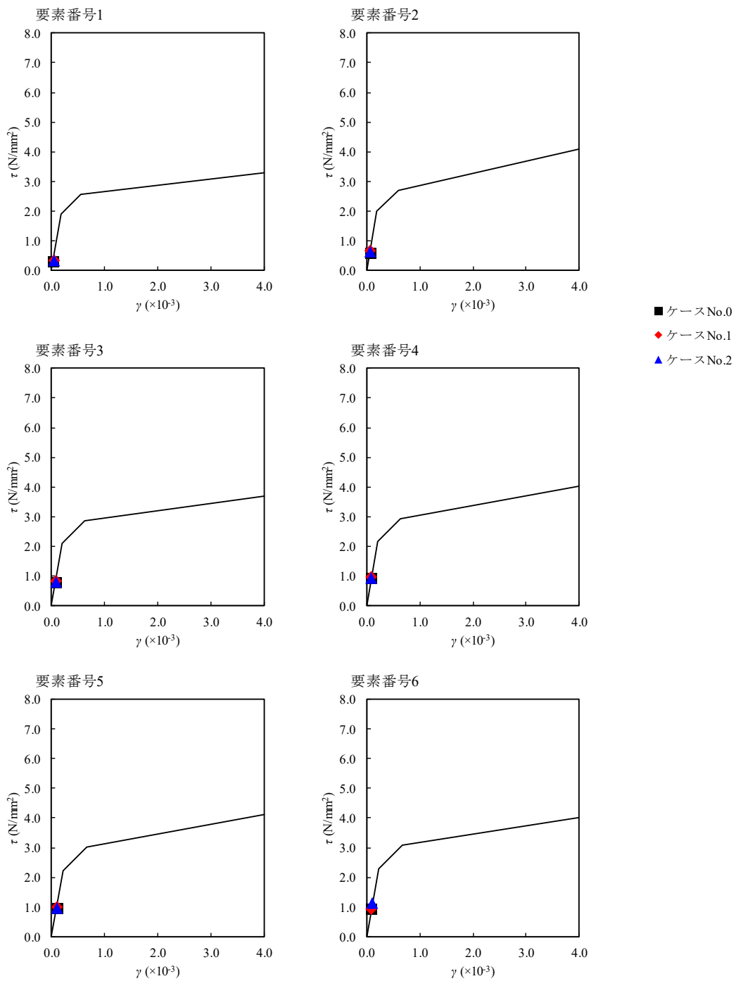
第 4.1.3-47 図 \tau - \gamma 関係と最大応答値 (S d - A, EW 方向)
