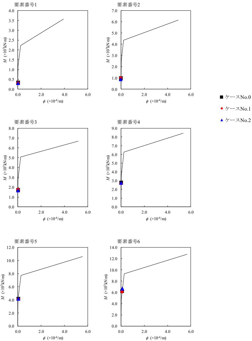
第 4.1.3-27 図 M- \phi 関係と最大応答値 (S s -C1, EW 方向)
