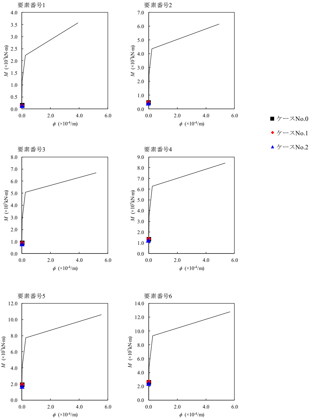
第 4.1.3-50 図 M- \phi 関係と最大応答値 (S d - B 1, EW 方向)
