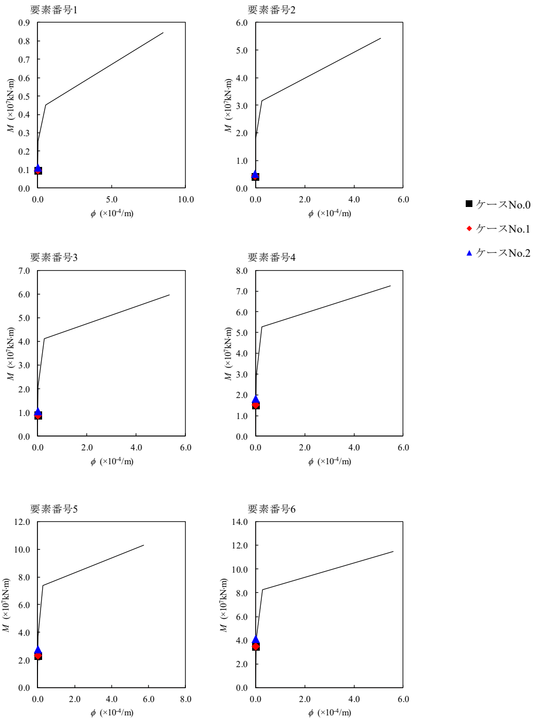
第 4.1.3-46 図 M- \phi 関係と最大応答値 (S d - C 1, NS 方向)
