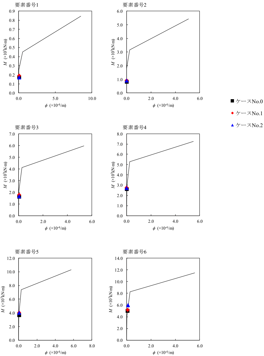
第 4.1.3-13 図 M-φ 関係と最大応答値 (S s - A, NS 方向)
