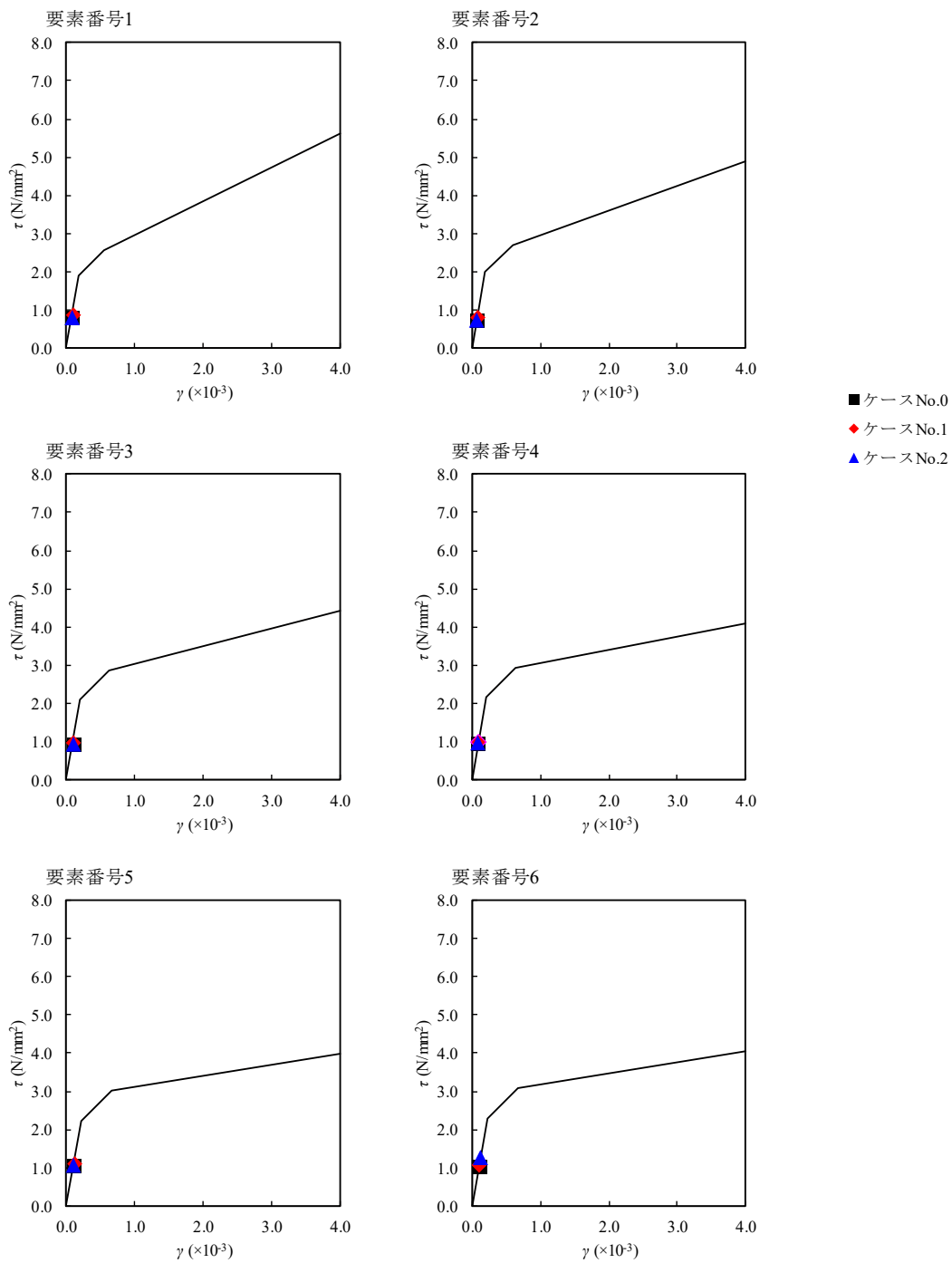
第 4.1.3-39 図 \tau - \gamma 関係と最大応答値 (S d - A, NS 方向)
