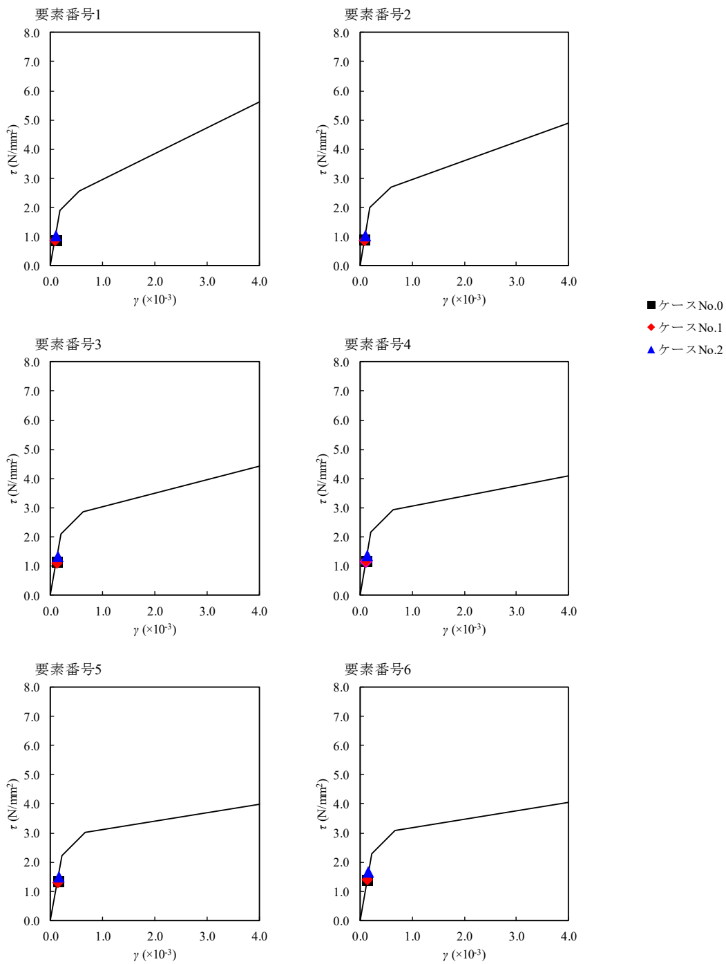
第 4.1.3-45 図 \tau - \gamma 関係と最大応答値 (S d - C 1, NS 方向)
