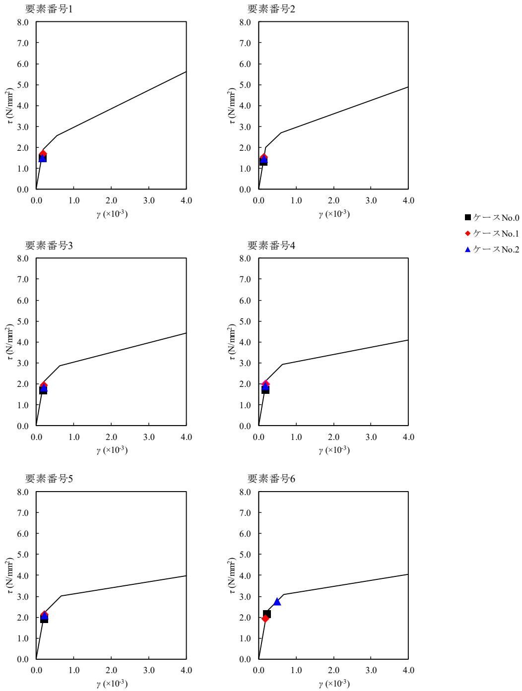
第 4.1.3-12 図 \tau - \gamma 関係と最大応答値 (S s - A, NS 方向)
