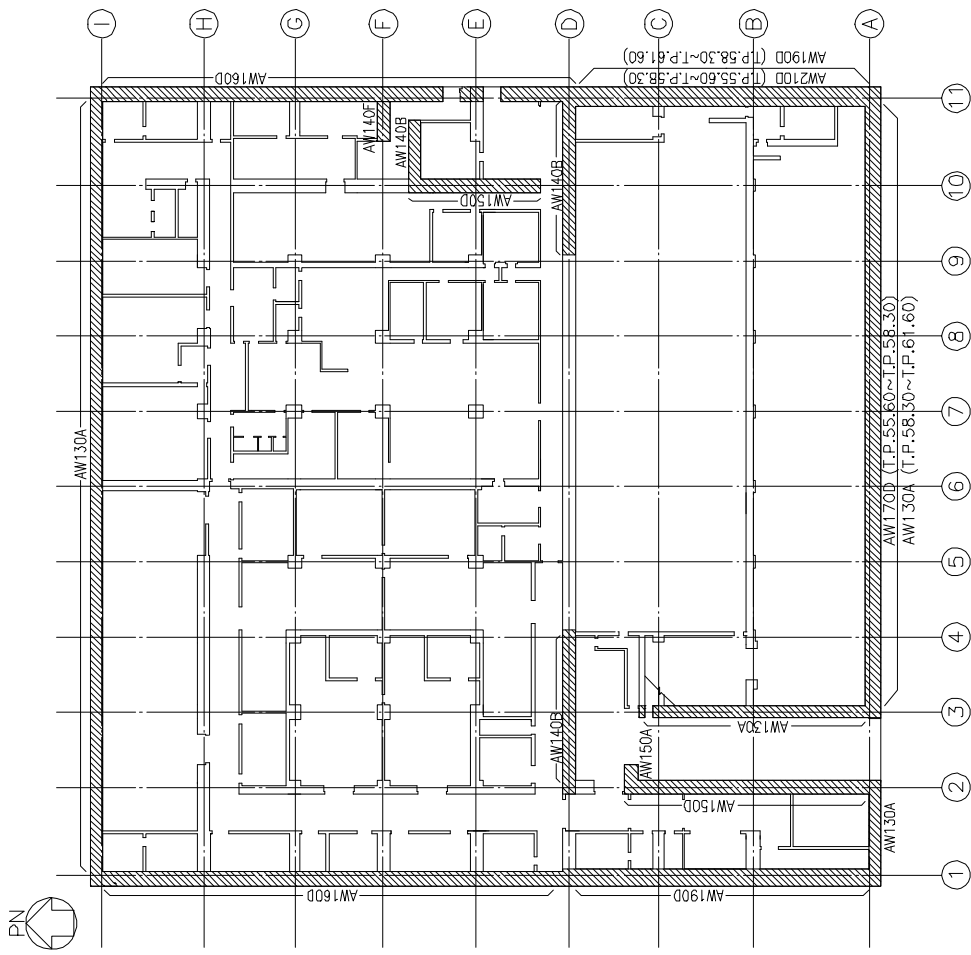
1階キープラン (T.P.55.60m) 注：[ハatched] は防壁を示す。
