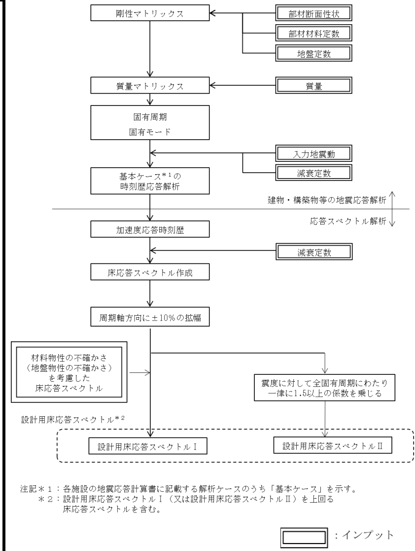
図 2-1 設計用床応答スペクトルの作成方法
