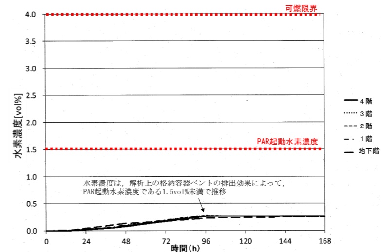
図 2-16 ケース 1 水素濃度の時間変化 (原子炉建物原子炉棟全
