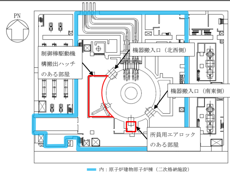
図 2-14 原子炉建物 1 階
