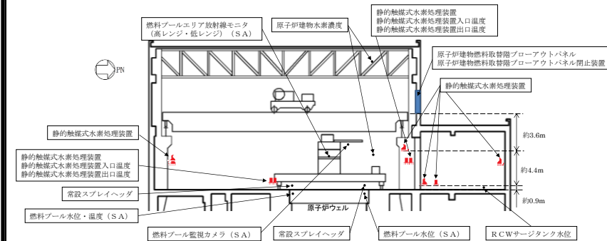
図 3-1 原子炉建物原子炉棟 4 階における重大事故等対処設備の機器配置 (1/2)
