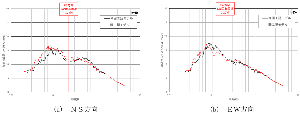
図 3-1 既工認モデルと今回工認モデルによる入力地震動の加速度応答スペクトルの比較 (原子炉建物, 基準地震動 S s - D)
