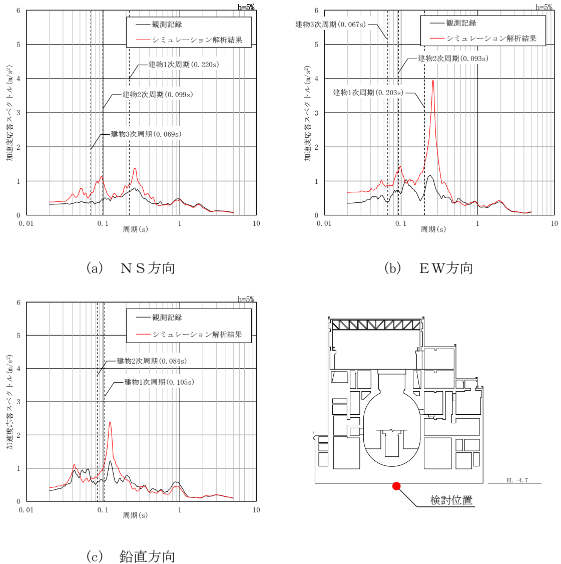
図 4-21 加速度応答スペクトルの比較
