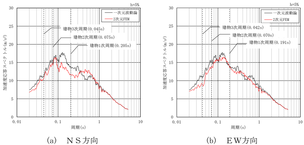
図 4-11 入力地震動の加速度応答スペクトルの比較 (廃棄物処理建物, 基準地震動 S s - D)
