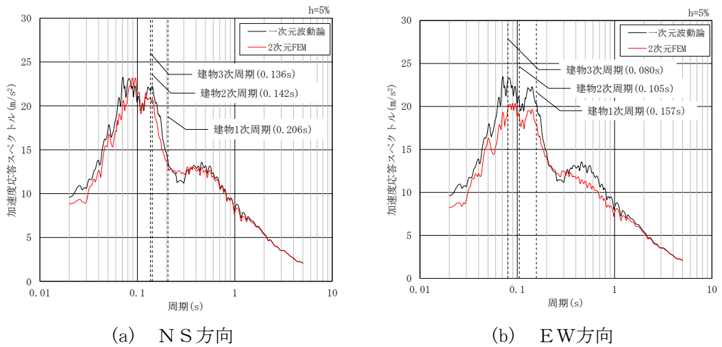
図 4-10 入力地震動の加速度応答スペクトルの比較 (タービン建物, 基準地震動 S s - D)
