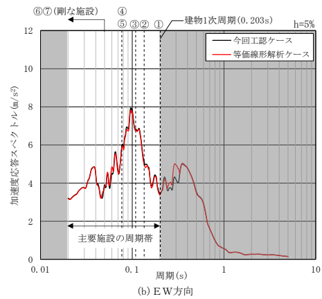
図 4-4(2) 入力地震動の加速度応答スペクトルの比較
