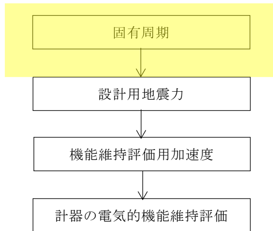
図 2-1 原子炉圧力容器温度（S A）の耐震評価フロー
