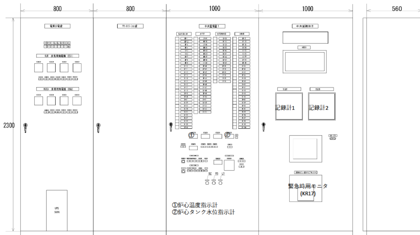
電源分電盤
