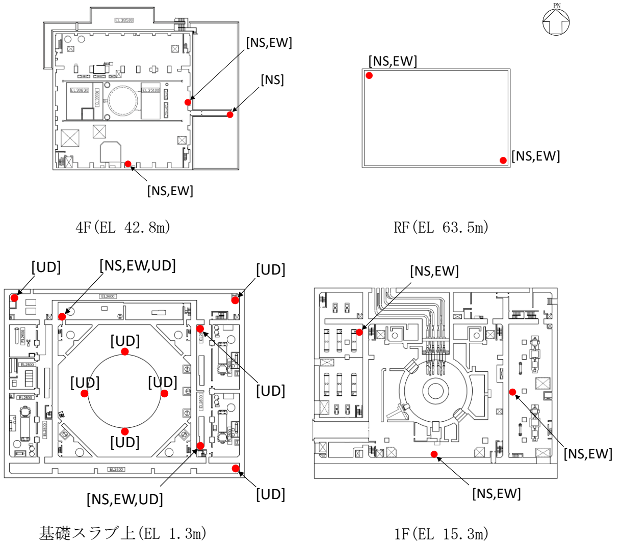
(1) 平面図
