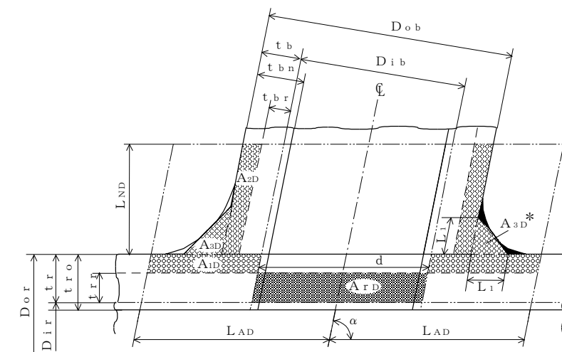
図 2-9 A形 (平板で強め材のない場合)
