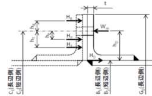
図 2-2 フランジの寸法 (矩形ダクト)
