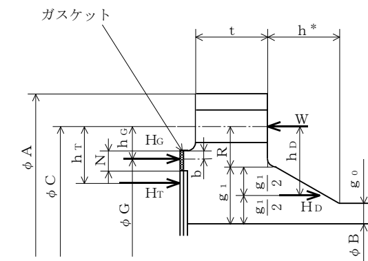
TYPE-5 JIS B 8265 附属書3 図2 b) 8)
