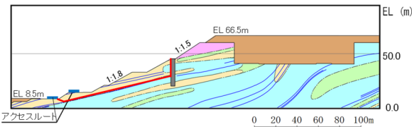
【B21・22シームを通り法尻に抜ける杭の肌別れを想定したすべり面】
