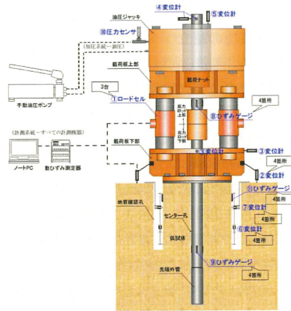
図 2.7.4-23 試験装置の概要
