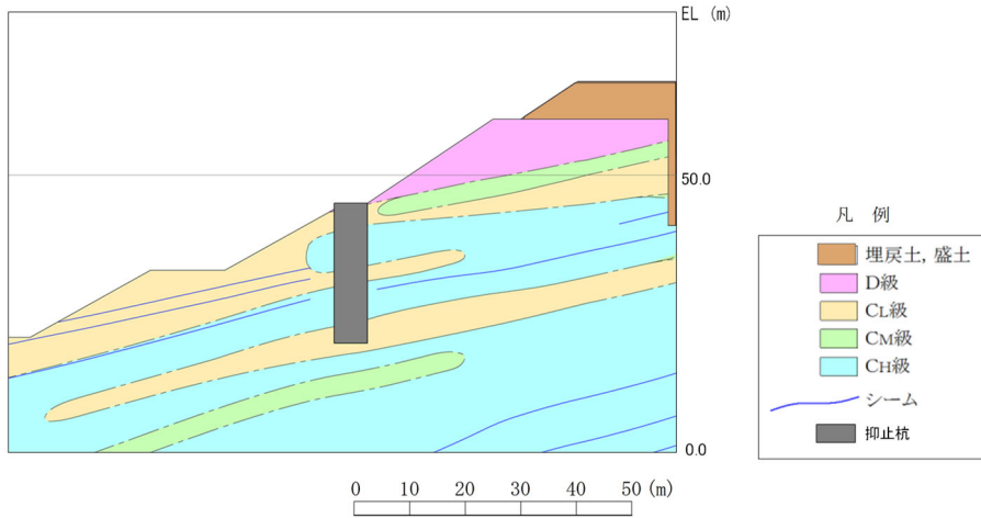
図 2.7.4-15 岩級区分図 (②-②' 断面)
