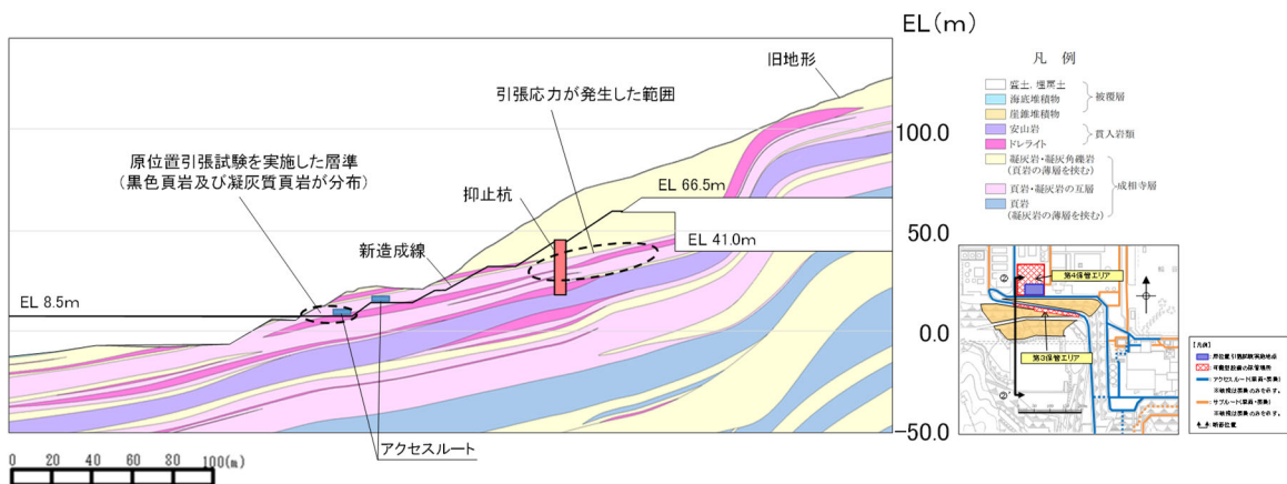
図 2.7.4-24 試験位置周辺の地質断面図
