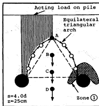
アーチ効果イメージ図 (文献④から抜粋)
