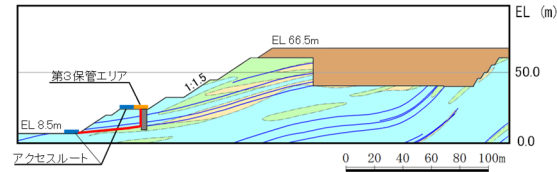
【B21シームを通して法尻に抜ける杭の肌別れを想定したすべり面】
