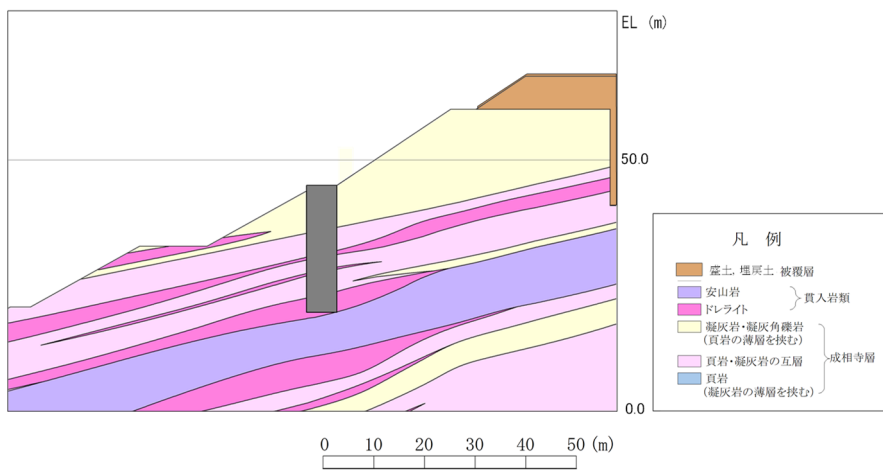
図 2.7.4-16 岩相区分図 (②-②' 断面)
