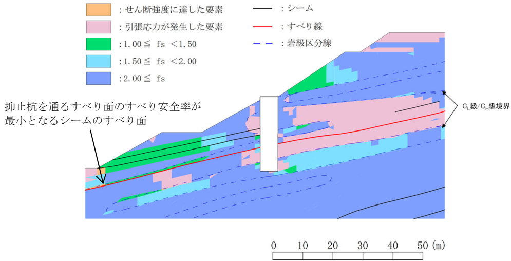
図 2.7.4-14 局所安全係数分布図 (②-②' 断面)
