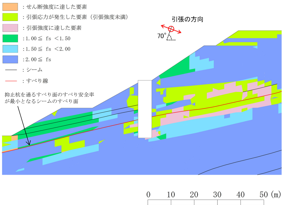
図 2.7.4-26 抑止杭周辺地盤の健全性照査結果 (②-②' 断面)
