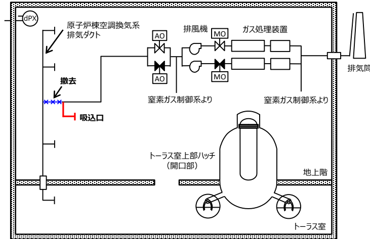
図1 非常用ガス処理系 系統概要図
