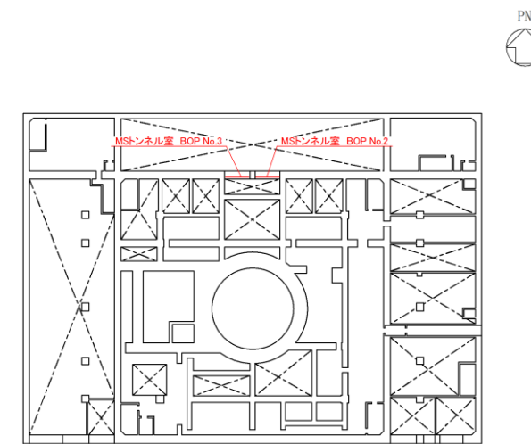
原子炉建物地上2階中間床 概略平面図
