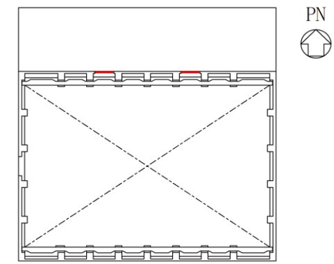
原子炉建物地上 4 階中間床 概略平面図 — (オペフロ BOP 2 箇所)
