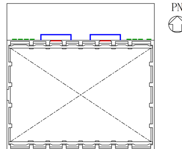
原子炉建屋地上4階中間床 概略平面図 : オペフロBOP : 竜巻防護ネット : 強制開放装置(保管箱)
