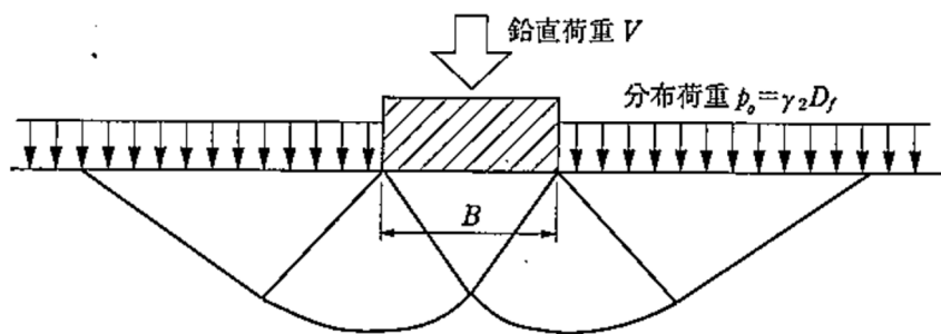
第5-3図 基礎の破壊時すべり線 (基礎指針2001)
