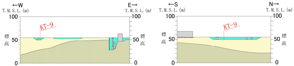
KT-9 断面
