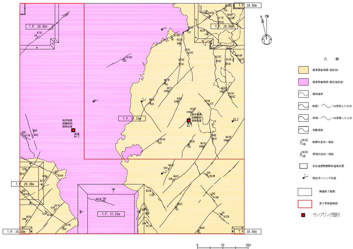
第5-2図 MOX燃料加工建屋直下掘削面の地質平面図及びサンプリング位置図
