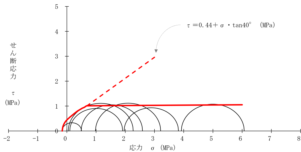
第 5-7 図 燃料加工施設の使用前検査における岩石強度試験結果（軽石凝灰岩）
