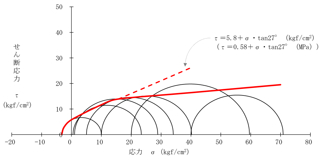
第 5-6 図 安全冷却水 B 冷却塔の使用前検査における岩石強度試験結果（細粒砂岩）
