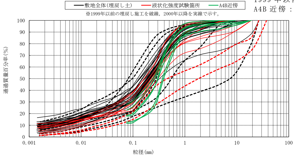
第 4-5 図 埋戻し土の粒度分布の比較
