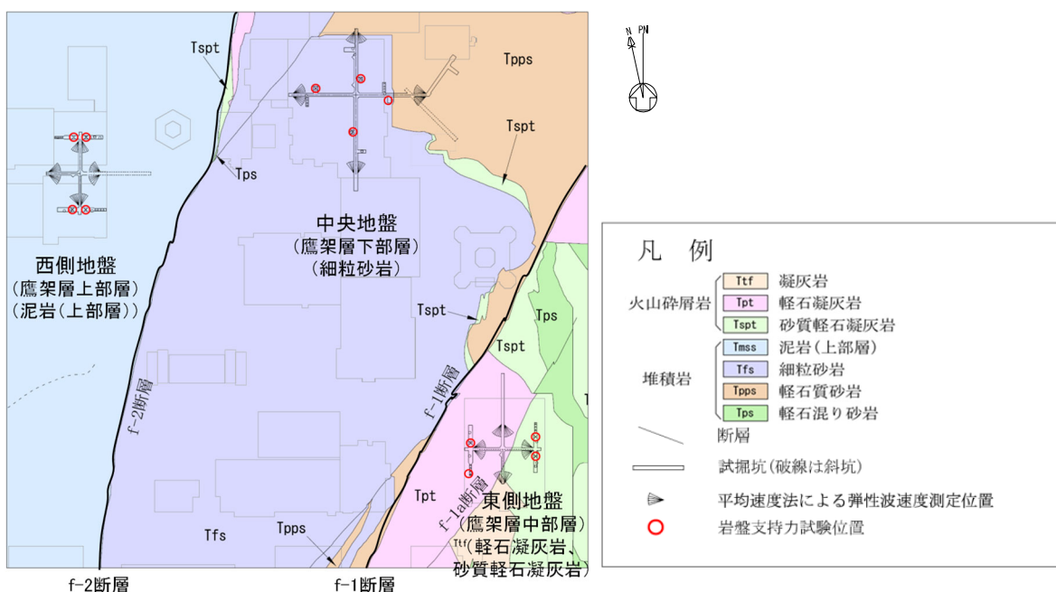
第 5-1 図 岩盤支持力試験位置図
