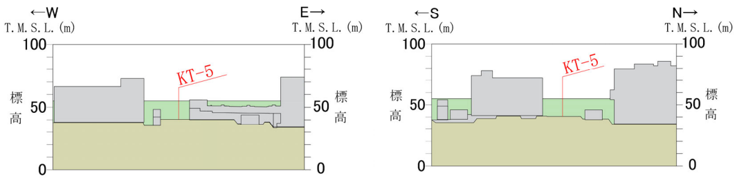
KT-5 断面
