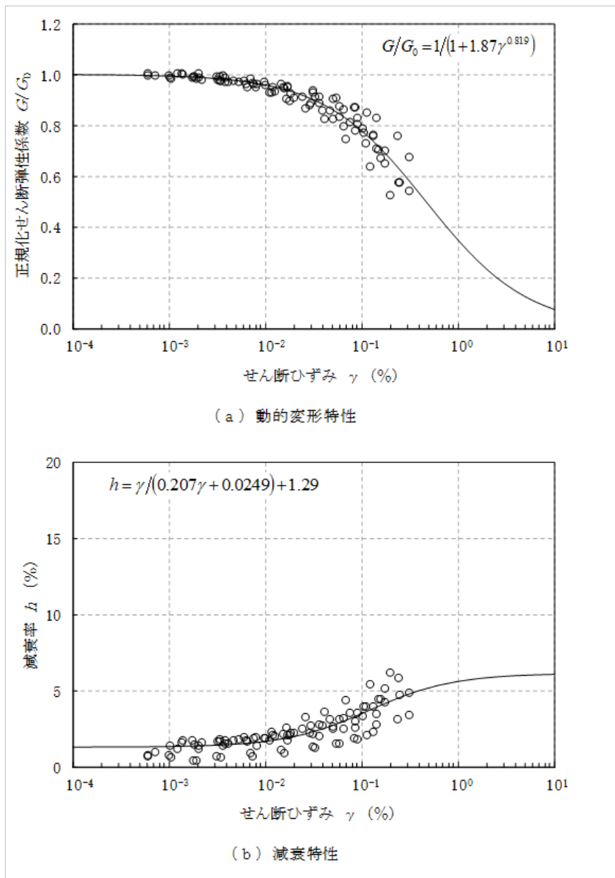
第 2.-3 図 細粒砂岩のひずみ依存特性 (「耐震建物 08 地震応答解析における地盤モデル 及び物性値の設定について」の別紙 1-1 第 2.1.2-3 図の再掲)
