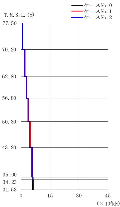
第 4.2-22 図 最大応答せん断力 (NS 方向) (1/2)
