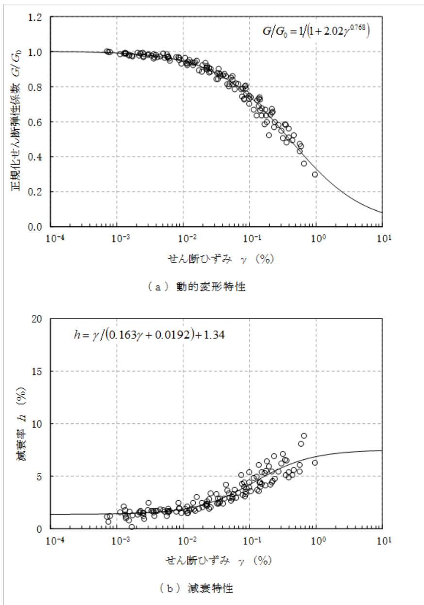
第 2.-1 図 軽石凝灰岩のひずみ依存特性 (「耐震建物 08 地震応答解析における地盤モデル 及び物性値の設定について」の別紙 1-1 第 2.1.2-1 図の再掲)
