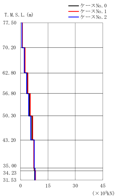
第 4.2-26 図 最大応答せん断力 (EW 方向) (1/2)
