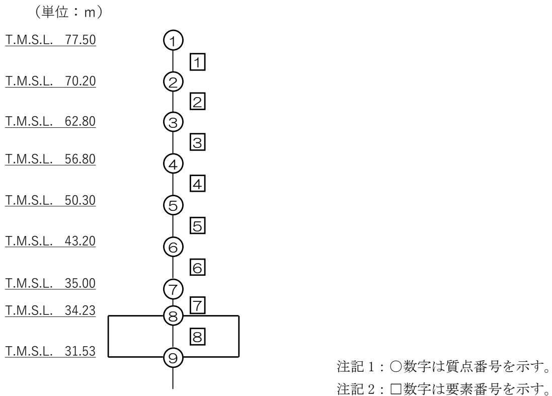
第 3.-1 図 建屋モデル
