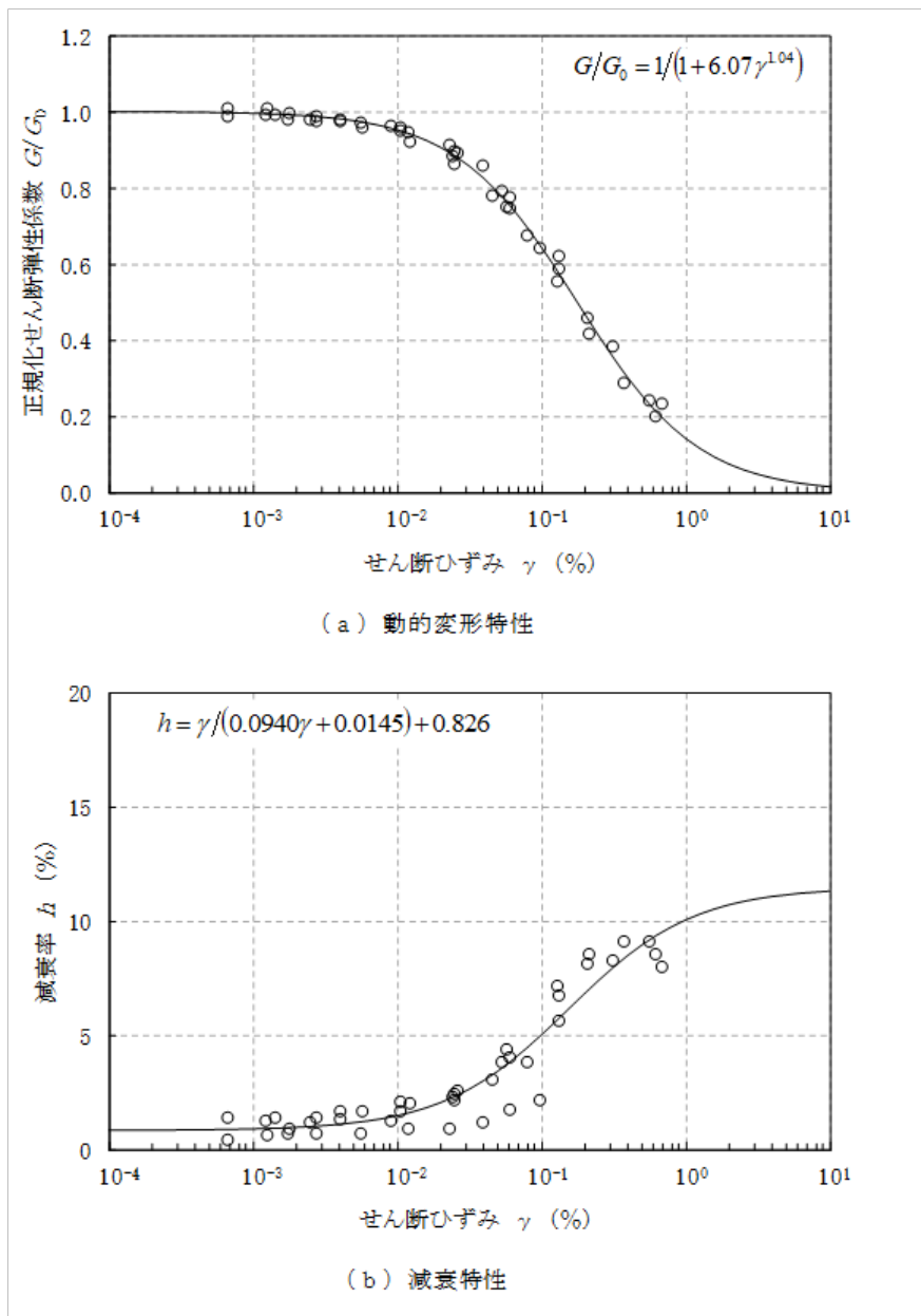
第 2.-2 図 軽石質砂岩のひずみ依存特性 (「耐震建物 08 地震応答解析における地盤モデル 及び物性値の設定について」の別紙 1-1 第 2.1.2-2 図の再掲)
