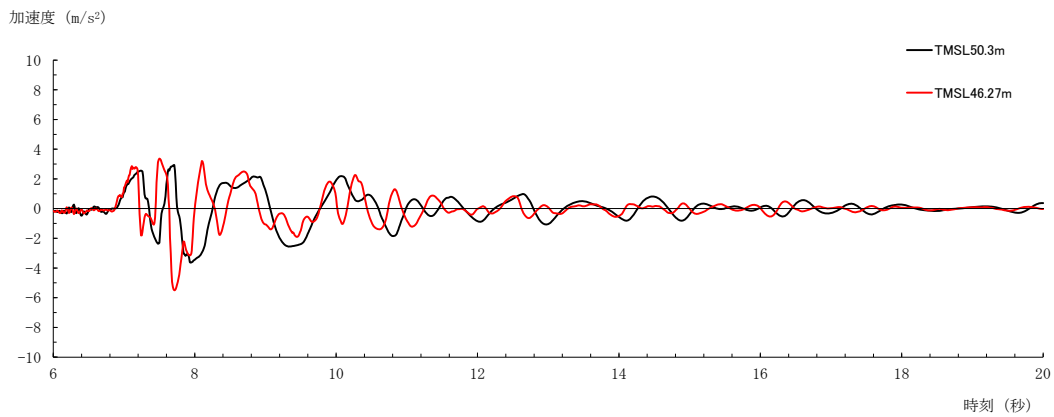
第 5.5-13 図 加速度時刻歴波形 ( S_s-C1 , -\sigma , 水平方向, 逐次非線形解析)
