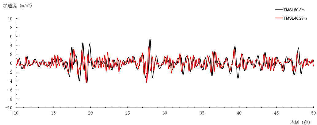
第 5.5-9 図 加速度時刻歴波形 (Ss-A, 基本, 水平方向, 等価線形解析) (10s~50s の範囲を切り出し, ハイカットフィルター (3Hz 以降))
