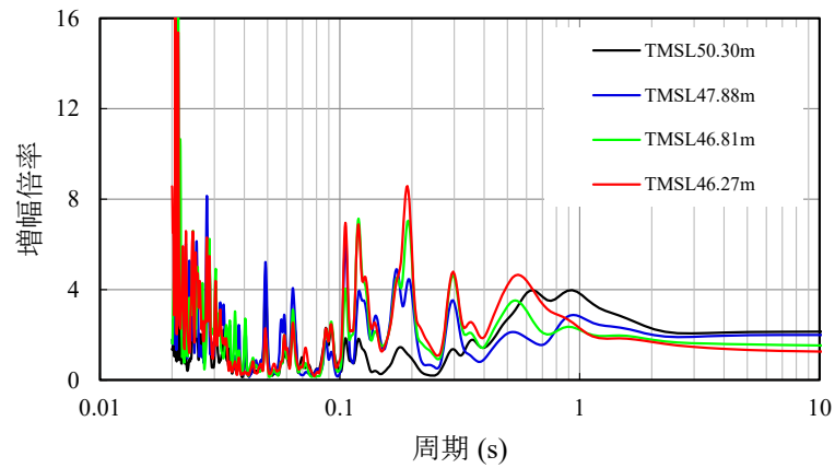
第 5.5-11 図 解放基盤表面に対する造成盛土のフーリエスペクトル比 ( S_s-C1 , -\sigma , 水平方向, 逐次非線形解析)
