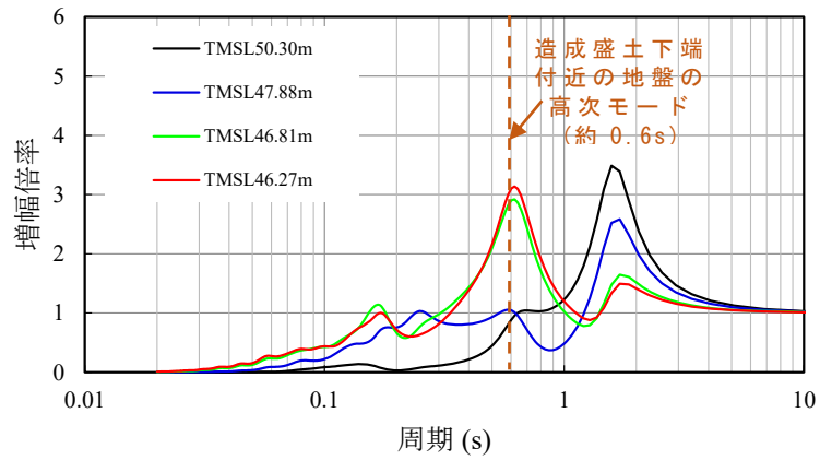
第 5.5-3 図 解放基盤表面に対する造成盛土の加速度伝達関数 (Ss-C1, -\sigma , 水平方向, 等価線形解析)
