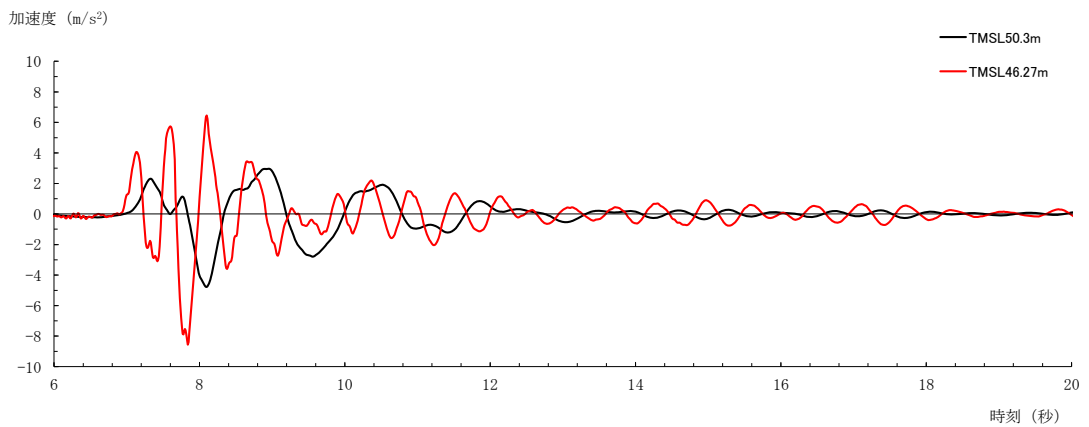
第 5.5-5 図 加速度時刻歴波形 (Ss-C1, -\sigma , 水平方向, 等価線形解析)
