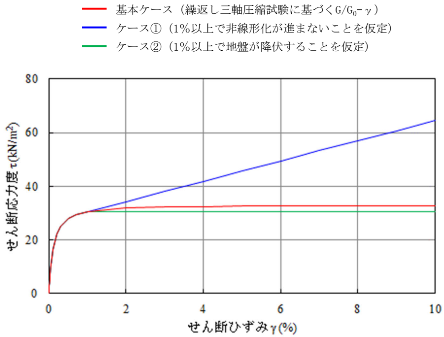
第 5.3-1 図 パラメータスタディにおいて考慮する地盤の骨格曲線
