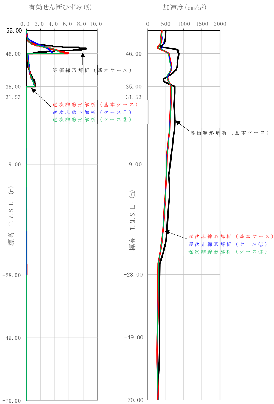
第 5.4-1 図 地盤応答分布図 S S -C1 ( - σ ) (逐次非線形解析)
