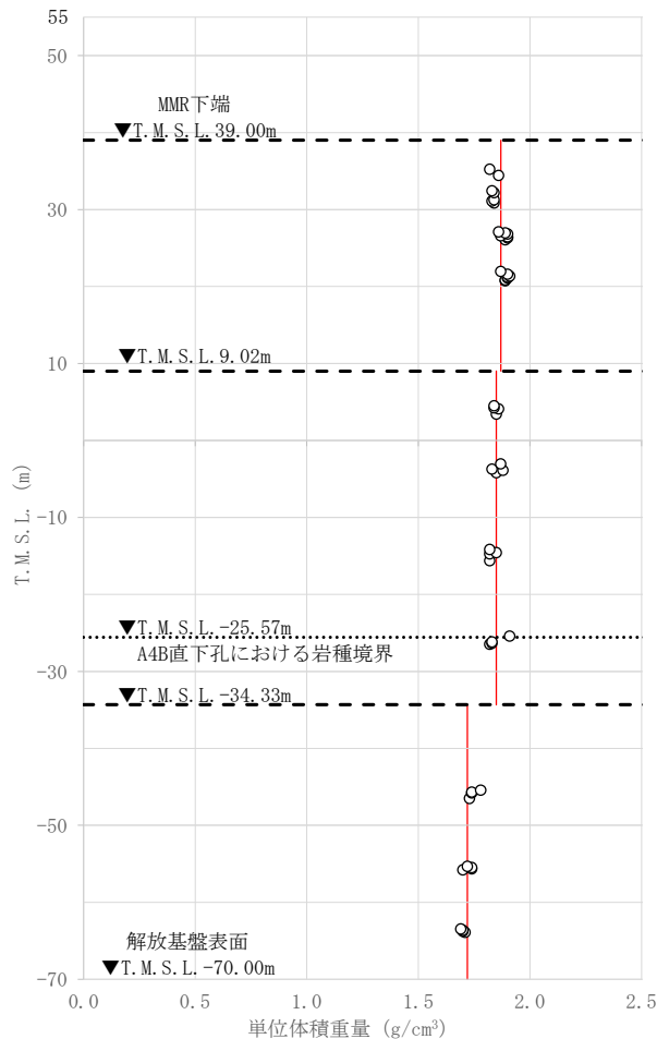
第 2.2-1 図 単位体積重量の設定結果
