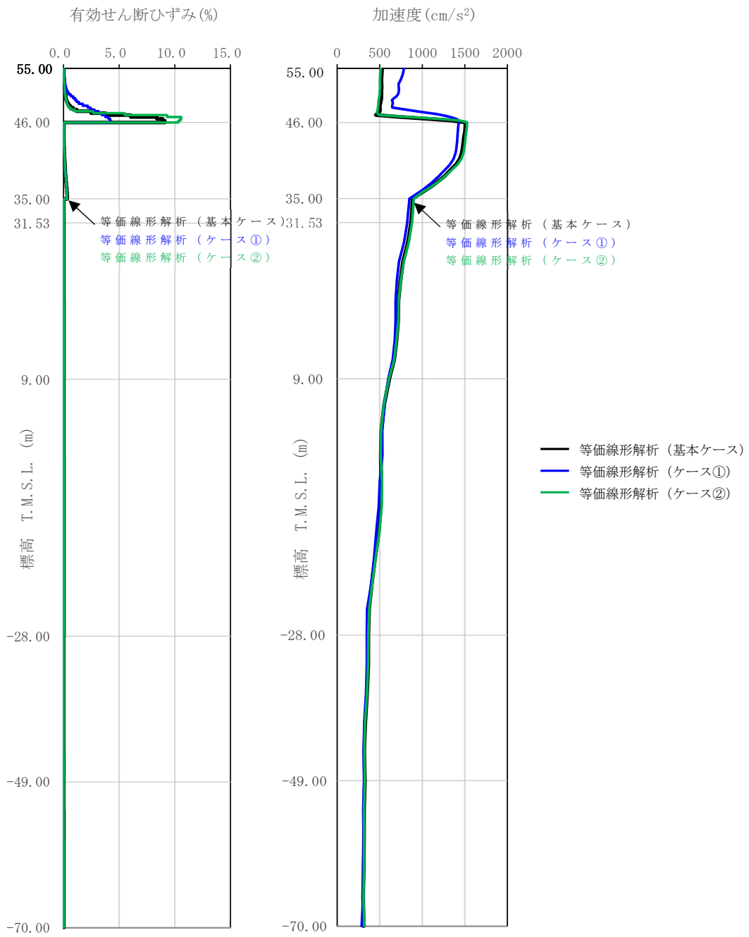
第 5.4-7 図 地盤応答分布図 1.2 \times S_s - C1 (等価線形解析)
