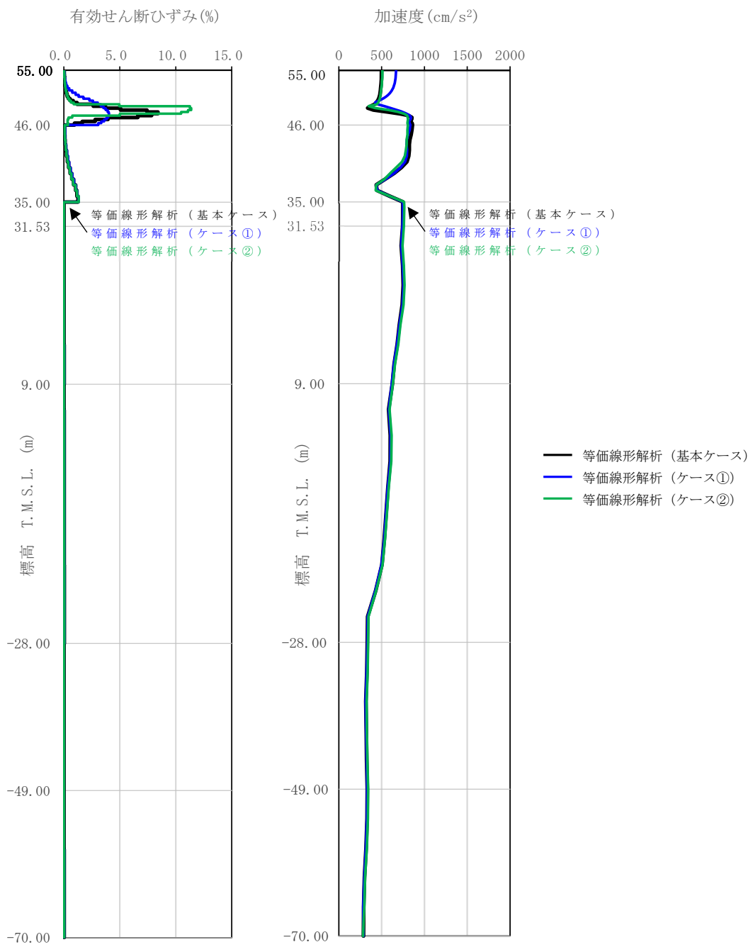
第 5.4-5 図 地盤応答分布図 S S -C1 ( - σ ) (等価線形解析)
