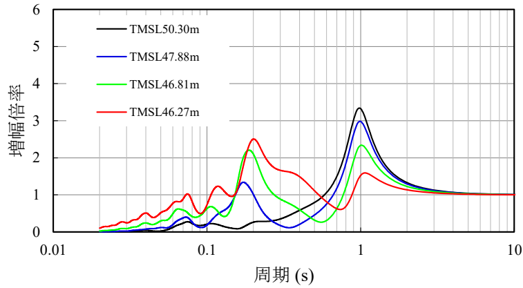
第 5.5-7 図 解放基盤表面に対する造成盛土の加速度伝達関数 (Ss-A, 基本, 水平方向, 等価線形解析)
