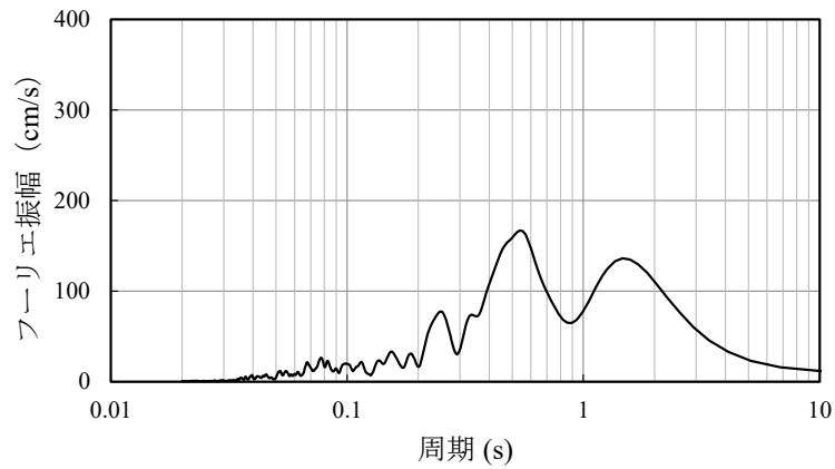
第 5.5-12 図 フーリエ振幅スペクトル ( S_s-C1 ) (Perzen ウィンドウ 0.5Hz)
