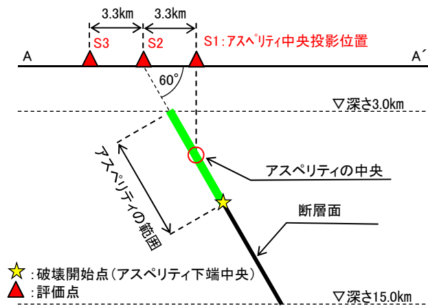
評価点の配置図(A-A'断面)
