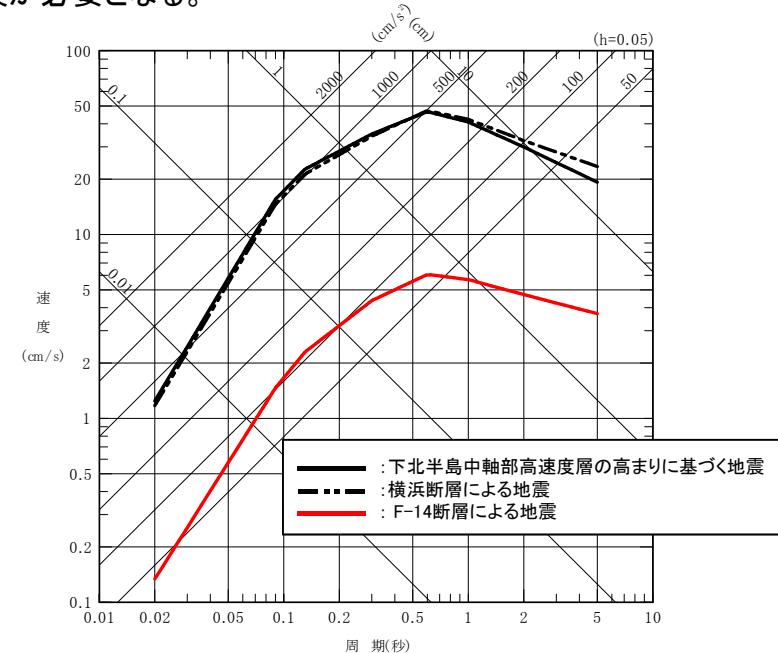
検討用地震及びF-14断層による地震の応答スペクトル 〔Noda et al.(2002), 水平方向, 内陸補正なし〕
