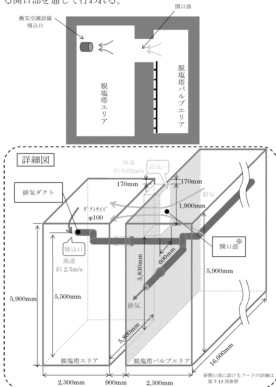
第 7-12 図 脱塩塔エリアの詳細図
