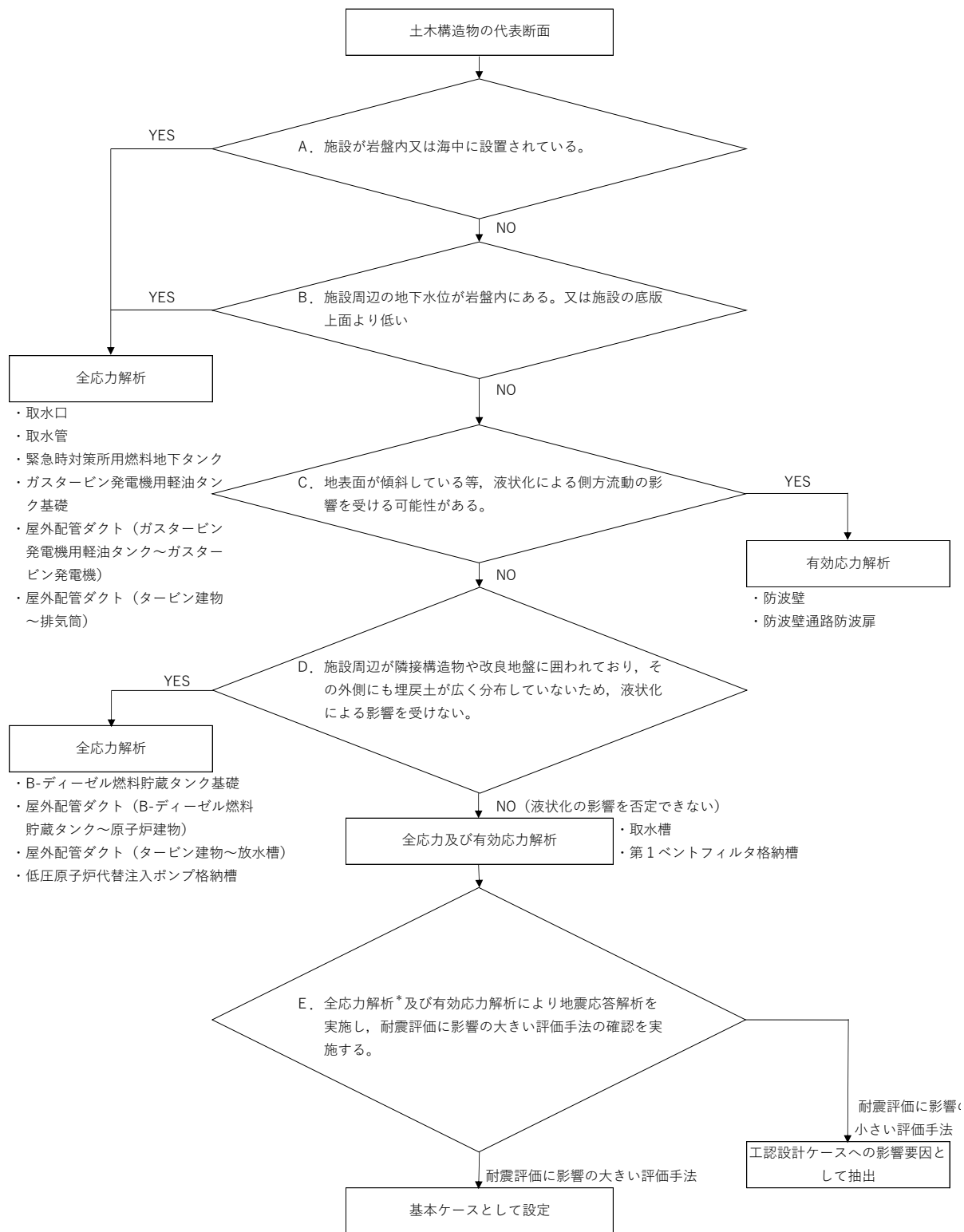
図 1(2) 島根 2 号機における地震応答解析手法の整理フロー（土木構造物）
