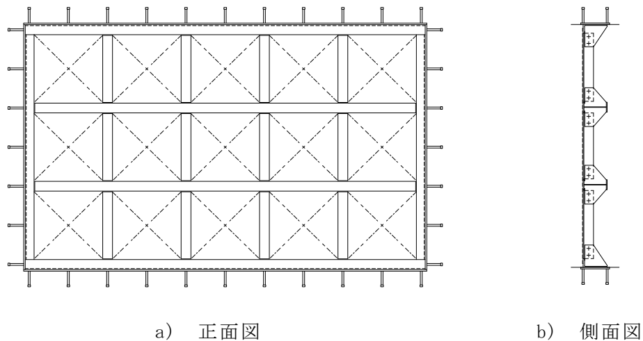
図 2-1 (1) 原子炉建物内側ブローアウトパネルの構造 (No.4, No.5 立面図)
