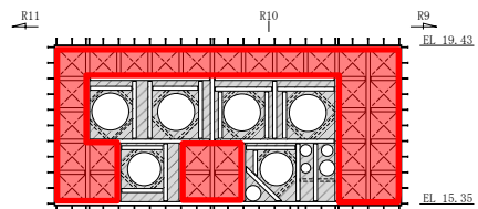
(a) MS トンネルBOP No. 1
