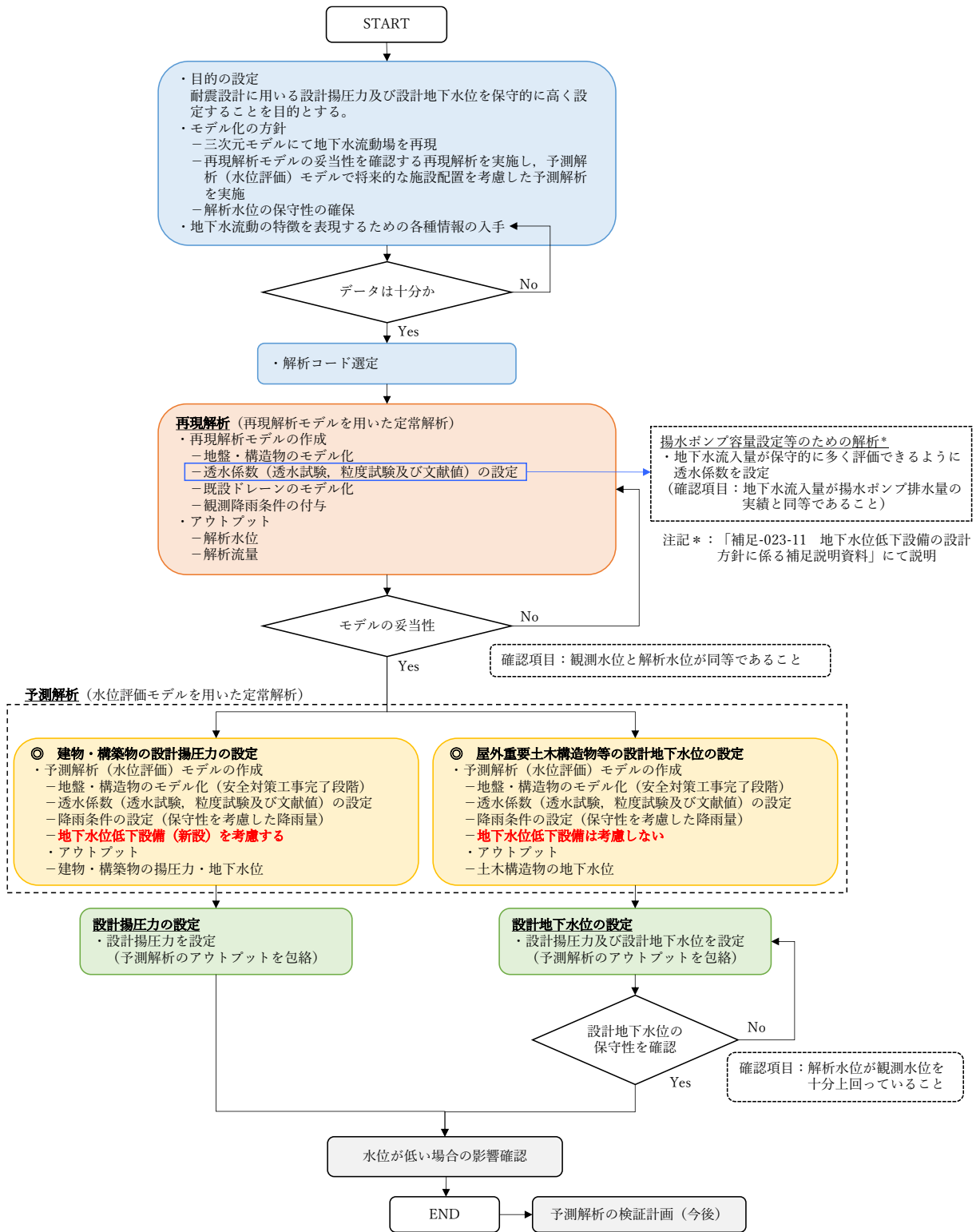
図 3.3-5 設計揚圧力及び設計地下水位の設定フロー
