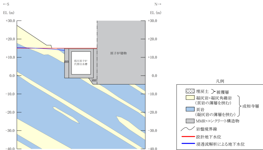
図 3.3-28 低圧代替注水ポンプ格納槽の地下水位分布(南北:水室)
