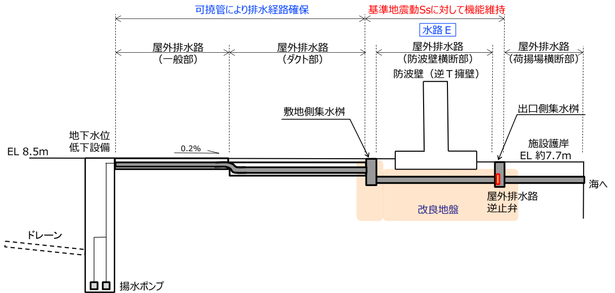
図 3-2 屋外排水路の耐震性の確保範囲
