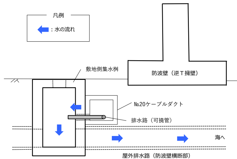
(4) C - C 断面
