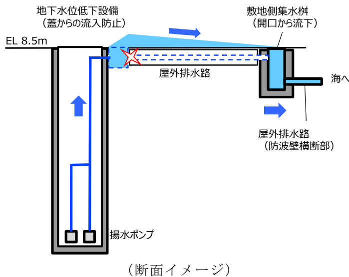
図 3-1 地表面を通じた排水の考え方
