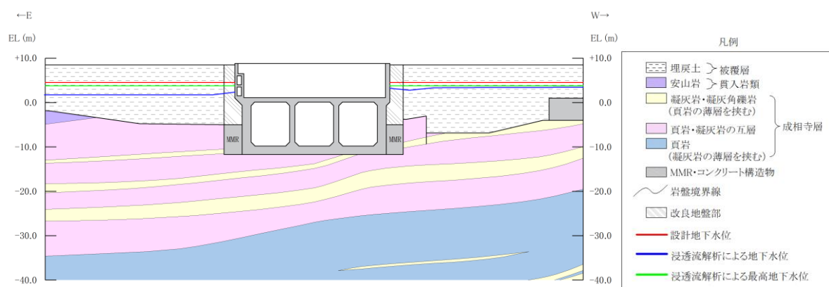
図 3.3-21 取水槽（ポンプ室）の地下水位分布
