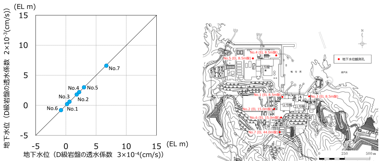
図 2-13 浸透流解析結果（地下水位）
