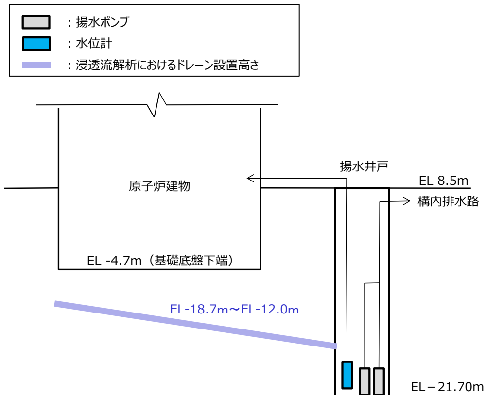
図 3-2 地下水水位低下設備（新設）の構成図
