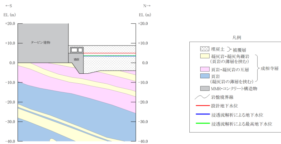
図 3.3-24 屋外配管ダクト（タービン建物～排気筒）の地下水位分布（横断）
