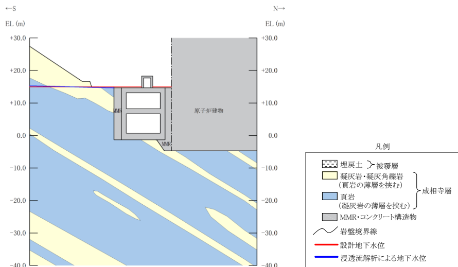
図 3.3-29 低圧代替注水ポンプ格納槽の地下水位分布(南北:ポンプ室)
