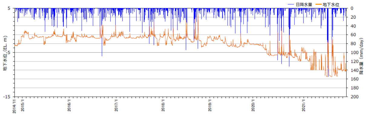
図 2-2(2) 地下水位観測記録 (No. 2 孔)
