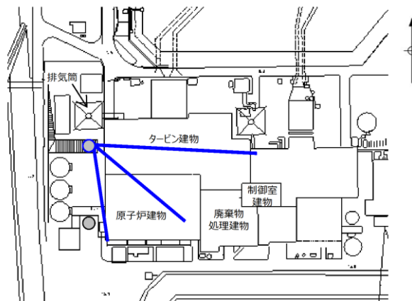
図3-1 地下水位低下設備（新設）の平面図
