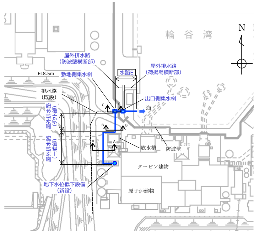
(1) 平面図
