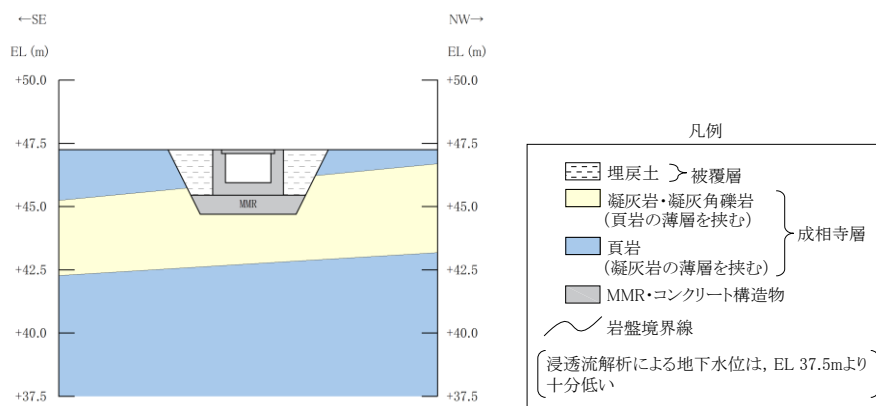
図 3.3-31 屋外配管ダクト (ガスタービン発電機用軽油タンク～ガスタービン発電機)の地下水位分布 (横断)
