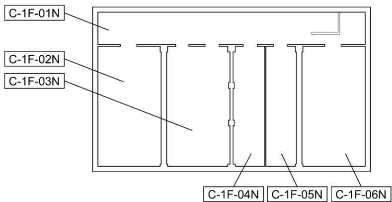
制御室建物 EL 1600
