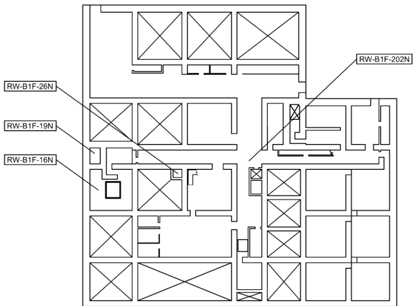
廃棄物処理建物 EL 3000
