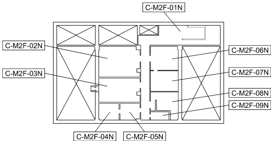
制御室建物 EL 5300
