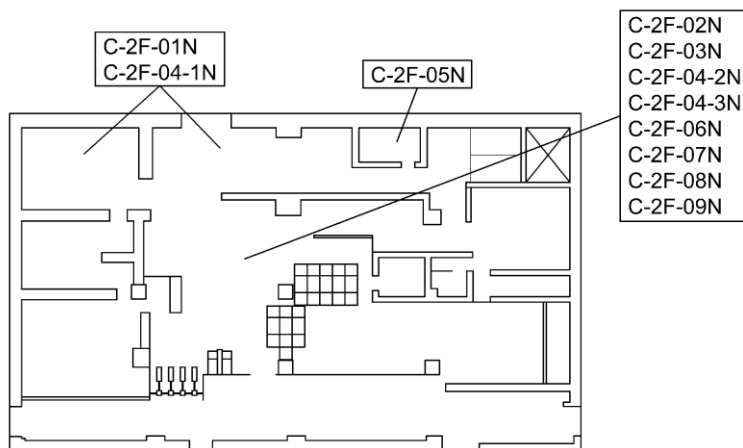
制御室建物 EL 5300
