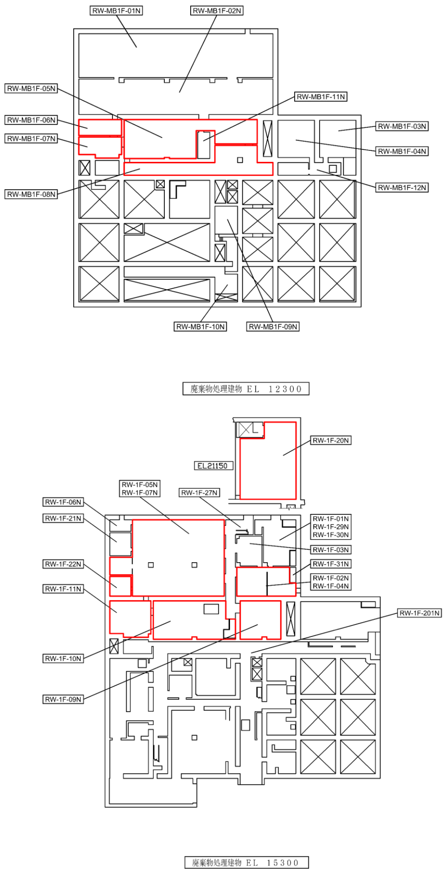
図 2-1 溢水防護区画 (6/14)
