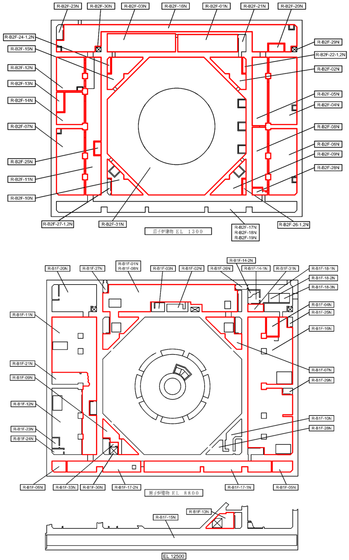
図 2-1 溢水防護区画 (1/14)
