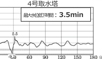
水位の時刻歴波形 ・朔望平均干潮位 T.P. - 0.93mを考慮
