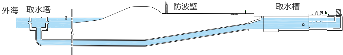
取水設備（取水塔～取水トンネル～取水槽）の縦断面図
