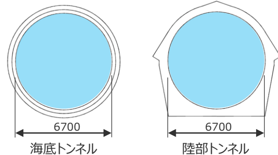
4号取水トンネル標準断面図
