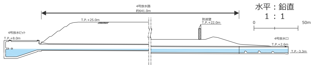
4号放水口～4号放水路～4号放水ピット縦断面図
