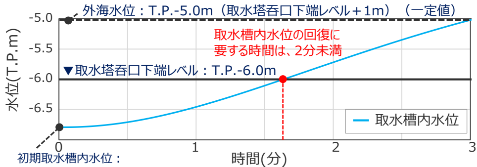
管路解析による取水槽内水位の時間変化
