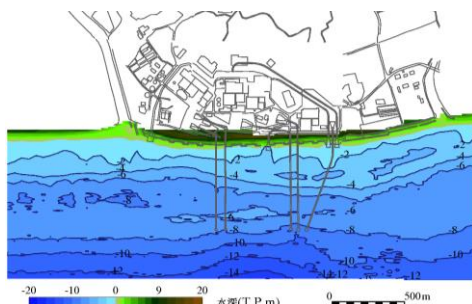
ケース2：運転時の単年地形 (2005月頃11月頃)
