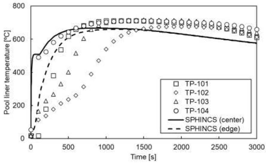
第 18 図 実験との比較 (燃烧皿ライナ温度、マルチセルプール燃烧実験)
