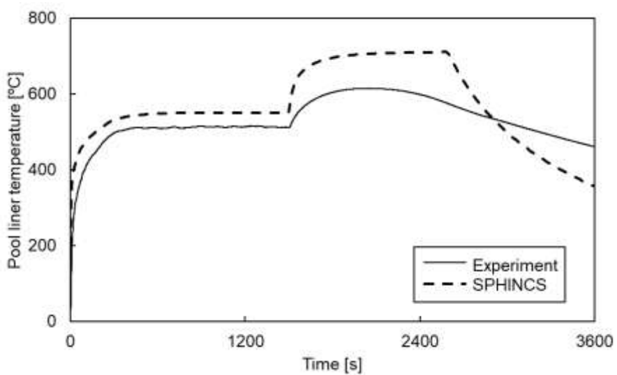
(c) プール下端ライナ温度時刻歴変化 (r=0.0m (center))
