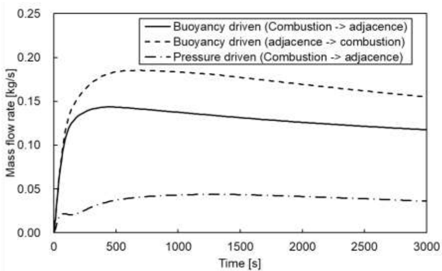
第 19 図 部屋間通気量 (マルチセルプール燃烧実験)
