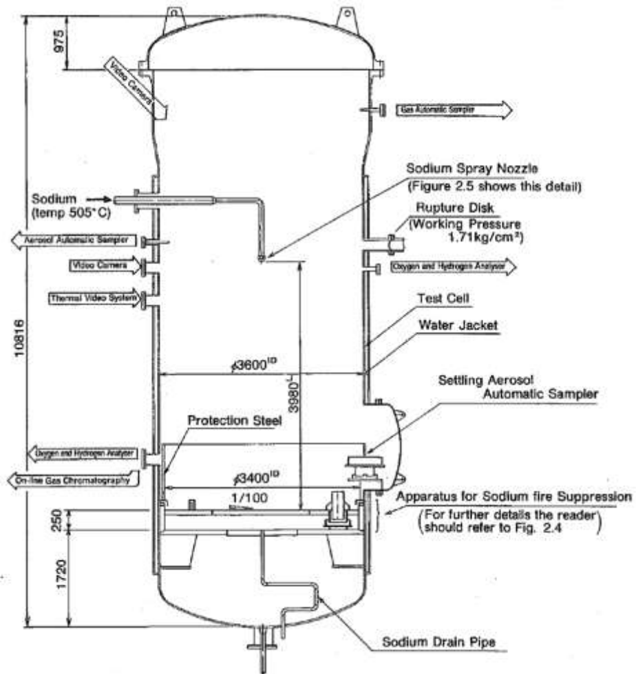
第 5 図 スプレー燃焼実験装置
