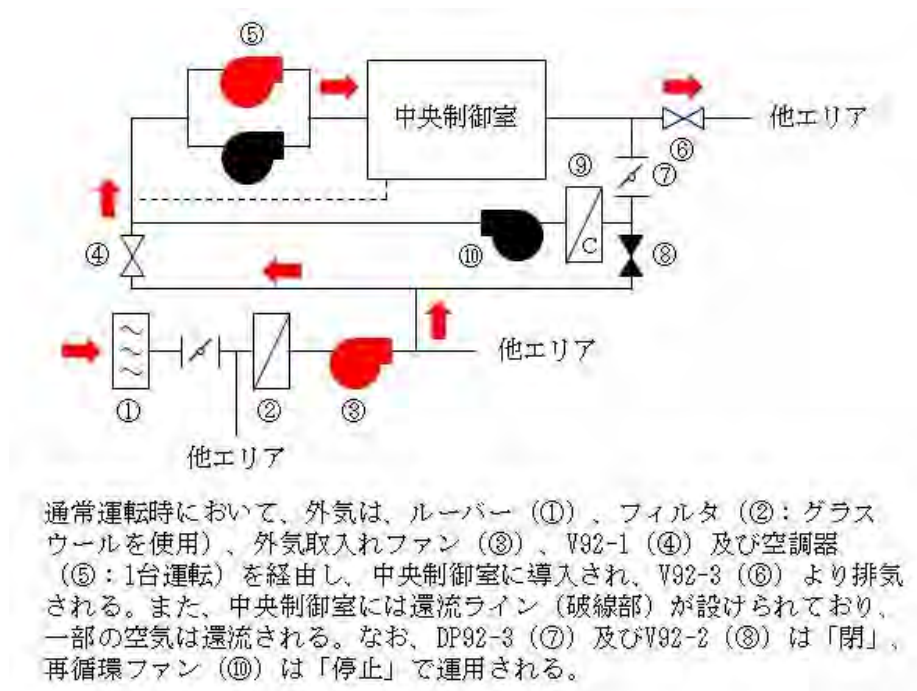
第1図 中央制御室空調換気設備の構成
