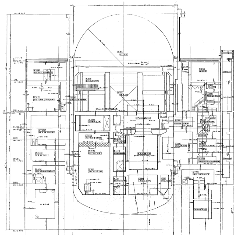
NS 断面
