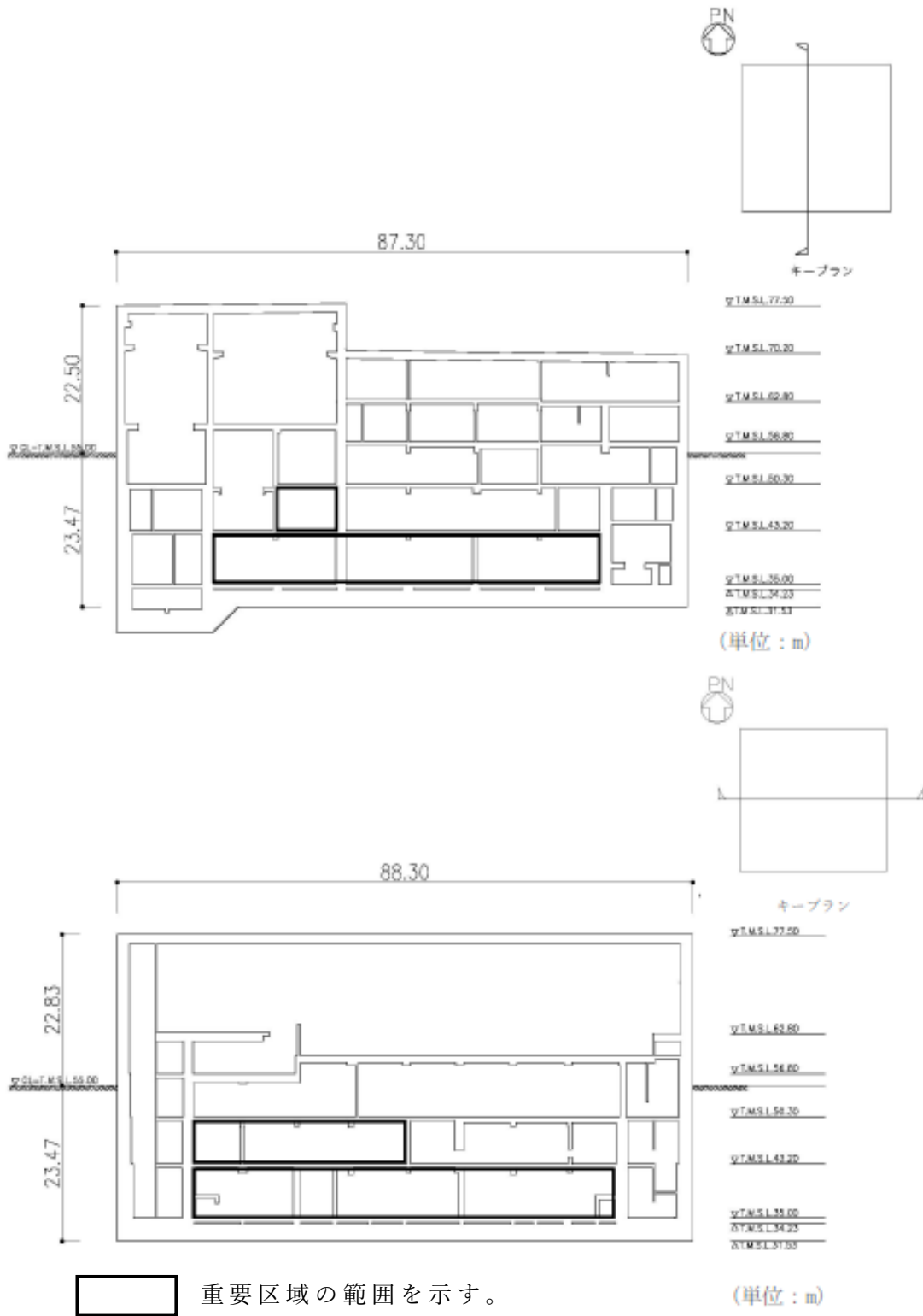
第 2.2.4-3 図 重要区域の範囲（燃料加工建屋の概略断面図） 【上：NS 方向，下：EW 方向】
