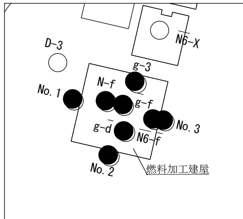
第3.-2図 地盤モデルの設定に用いるボーリング調査位置 (燃料加工建屋)
