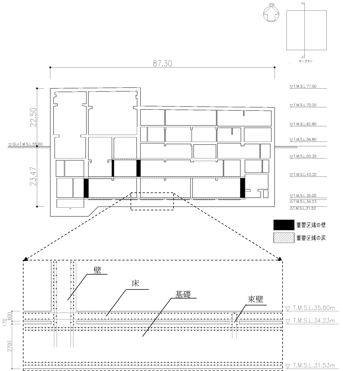
第 3.2-1 図 二重床部の詳細断面図
