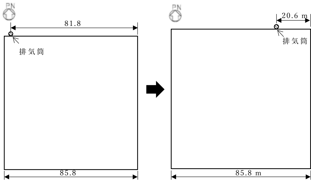
変更前 変更後 第 2.2.1-1 図 排気筒の位置変更
