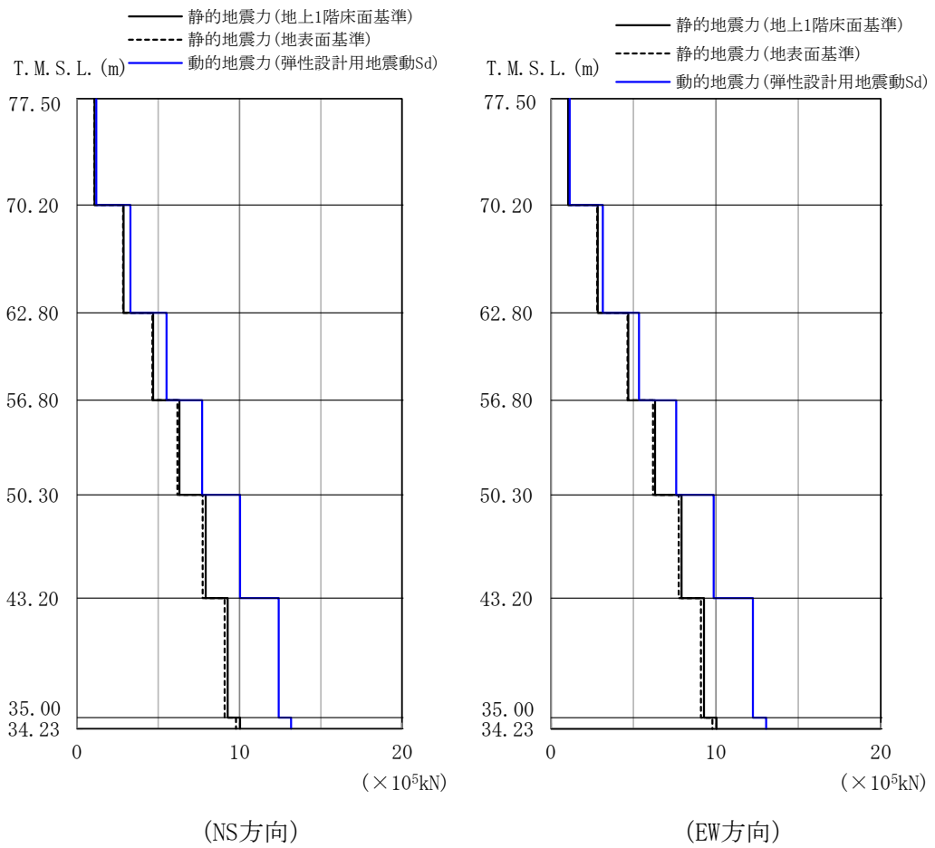
第3.-3図 静的地震力(地上1階床面基準, 地表面基準)及び動的地震力(弾性設計用地震動Sd)の比較
