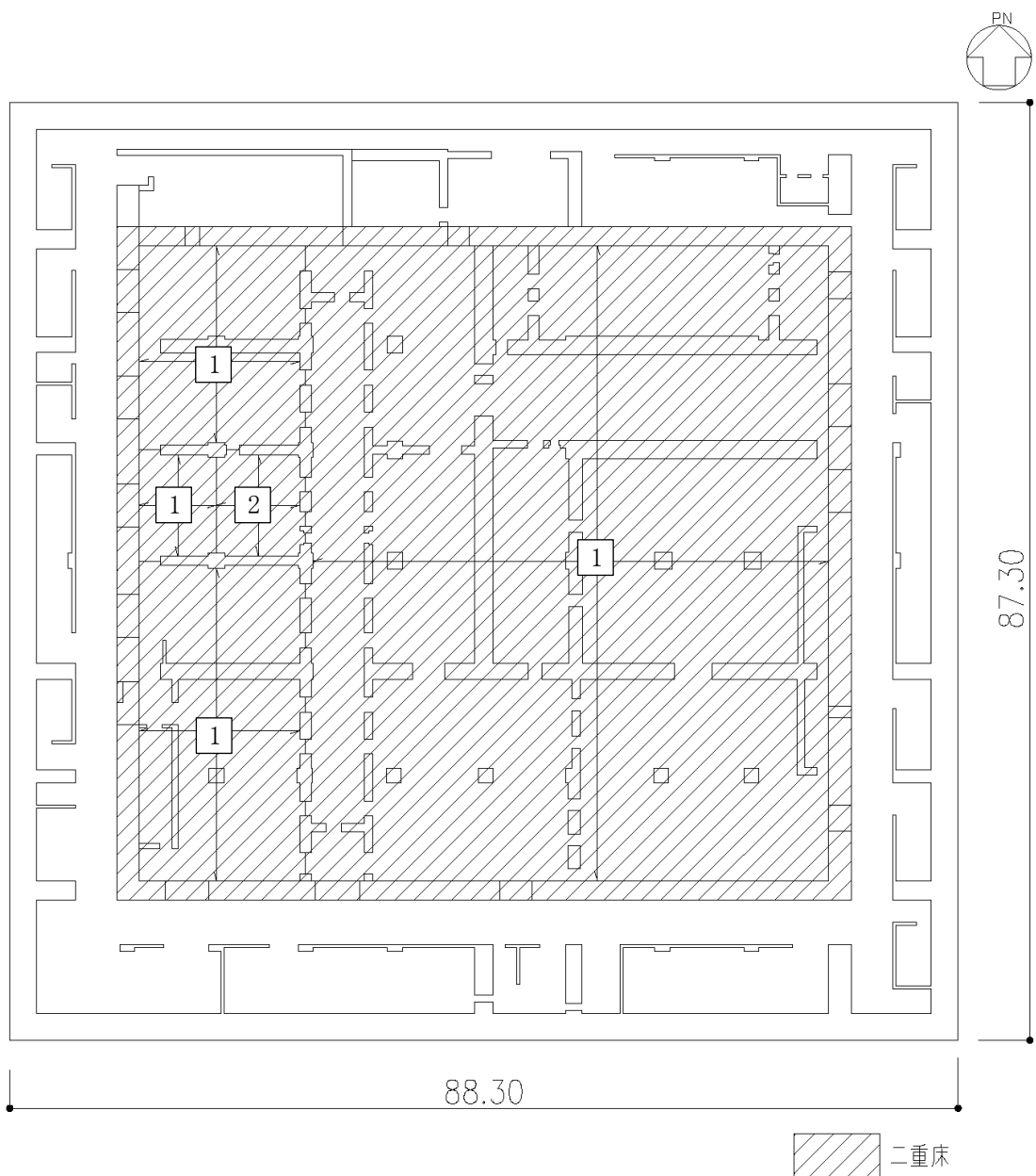
第 3.2-3 図 二重床の部材リスト (T. M. S. L. 35.00m)
