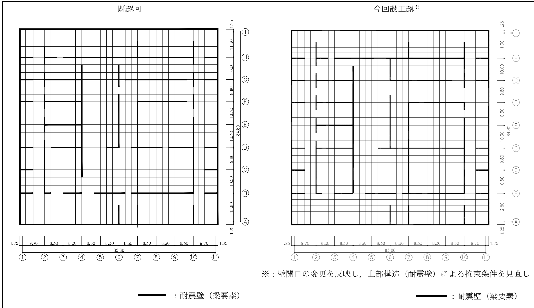
第 4. -1 図 応力解析モデルにおける上部構造による拘束の変更
