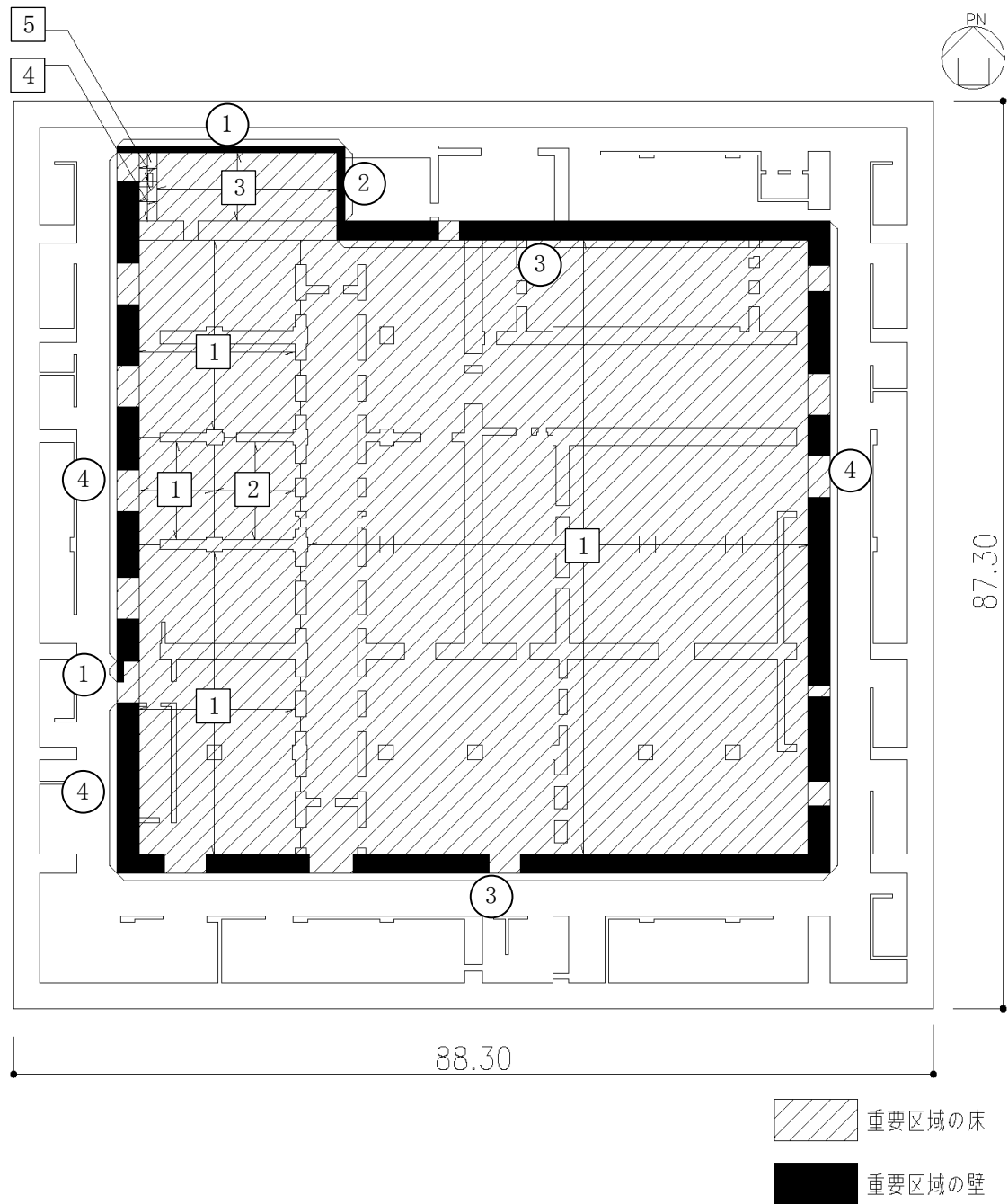
第3.1-1図 地下3階の部材リスト
