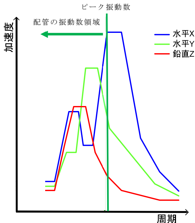
第2.2.4-1図 配管系の固有振動数とピーク振動数の関係
