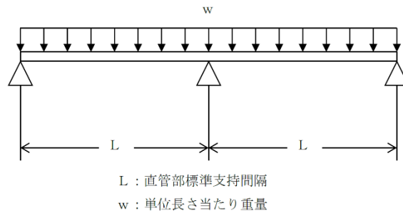
第2.2.2-1図 等分布荷重2スパン3点支持モデル
