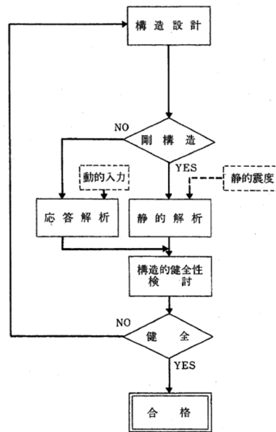
図6.7-4 電路類の耐震設計フローチャート
