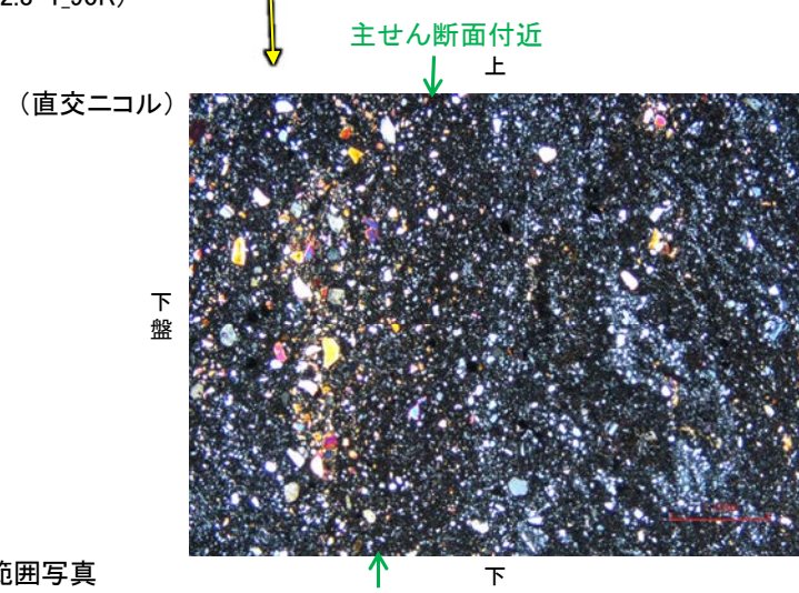
薄片写真(N-2.3-1_90R)
