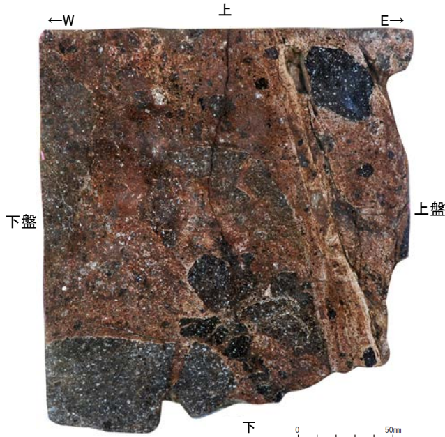
研磨片写真(右は変形構造を加筆) (薄片は研磨片の反対面で作成)
