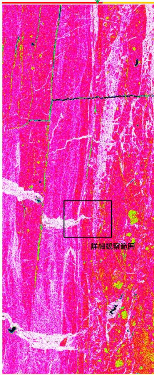
SiO 2
