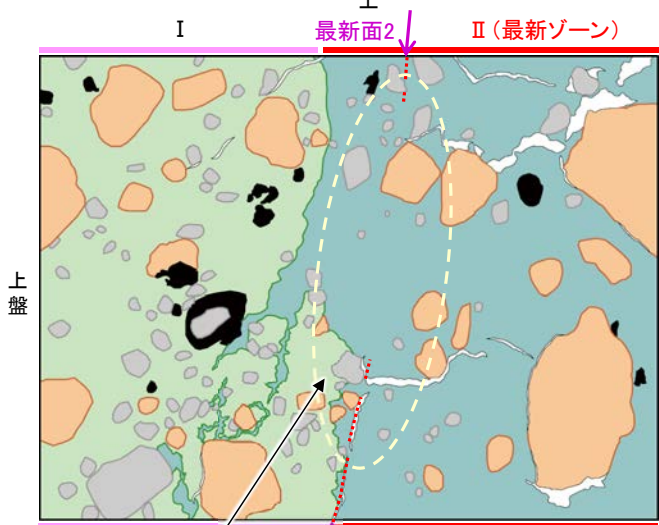
薄片①写真(H-6.6-1.71R)
