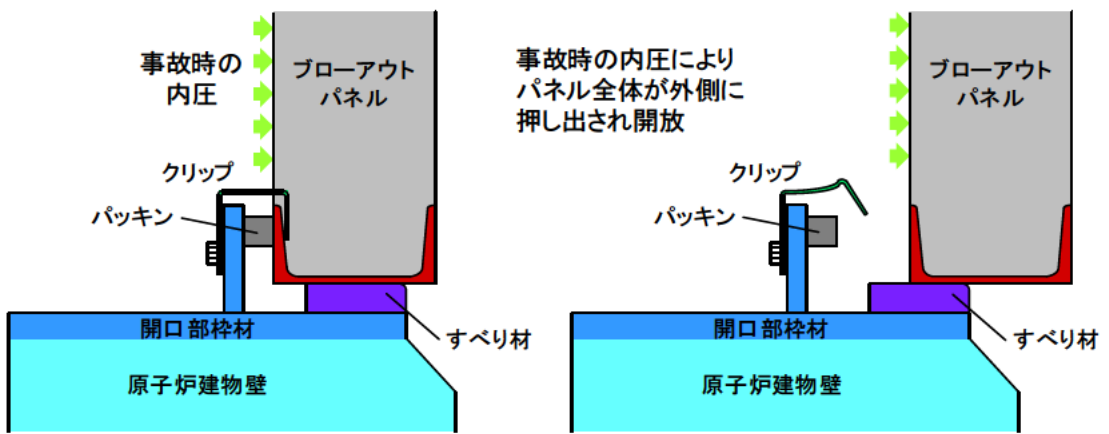
断面図（クリップ式構造の概念図）
