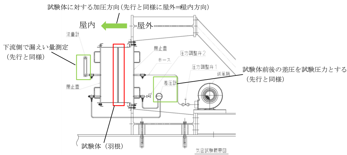
図 7-1 気密性能試験装置図
