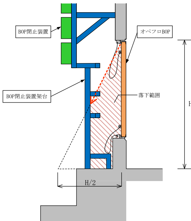
図 2-1 BOP 閉止装置架台図（断面図）
